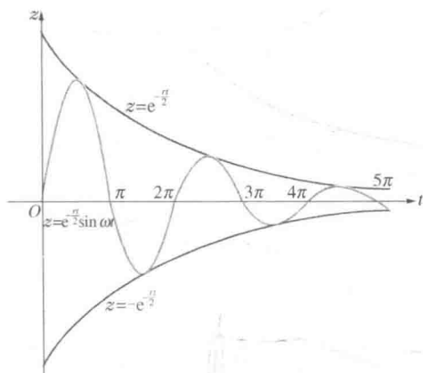
图 281 阻尼振动
