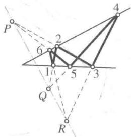
图 88 帕斯卡图形
