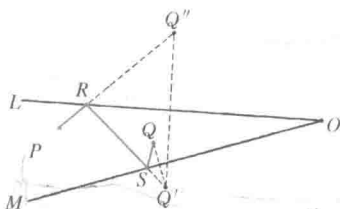
图 178 两镜面之间的反射
