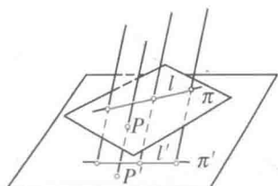
图 71 平行投影
