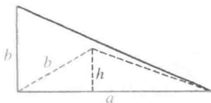
图 176
