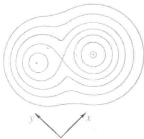
图 162 上图中相应的等高线
