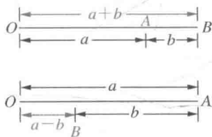
图 27 a+b 和 a-b 的作图
