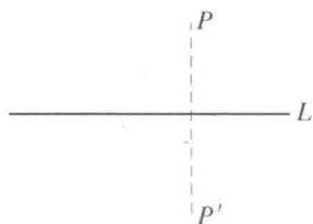
图 37 点对直线的反射
