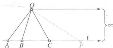
图 84 含有无穷远点的交叉比
