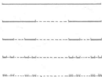
图 130 康托点集
