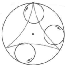
图 55 圆内三尖旋轮线
