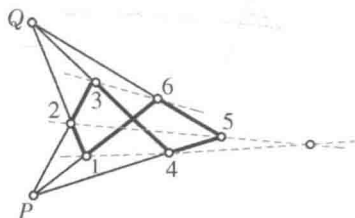
图 91 布利安桑图形
