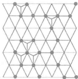
图 298
