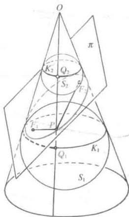
图 95 丹德林的球
