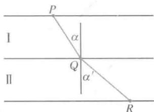
图 237 光线的折射
