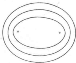
图 188 共焦点椭圆
