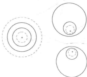
图 67 两个圆中的重复反射
