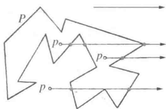
图 148 计算交点的个数
