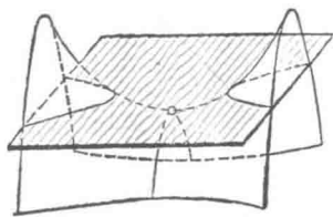
图 115 双曲点
