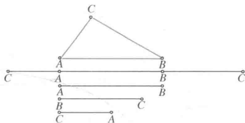
图 116 用标出端点的线段确定三角形
