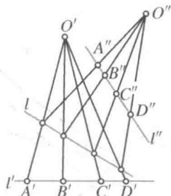
图 80 两条直线上的点的射影对应
