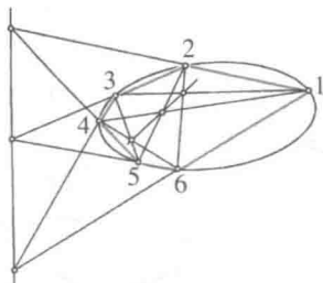
图 105 帕斯卡的一般图形 说明两种情形: 一个六边形是 1, 2, 3, 4, 5, 6. 一个六边形是 1, 3, 5, 2, 6, 4.
