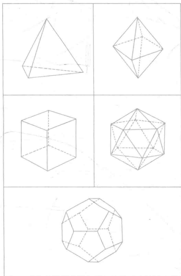
图 119 正多面体
