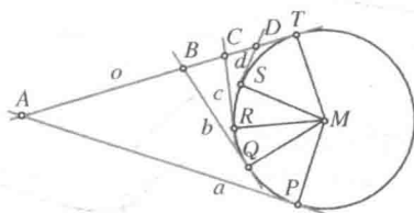
图 101 圆的切线性质
