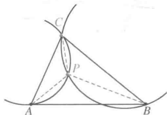
图 210
