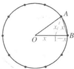
图32 正十边形
