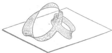
图 247 单围线内具有复杂拓扑结构的 单侧极小曲面
