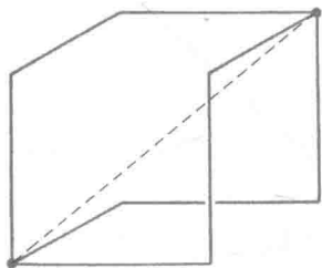
图 252 连接两点的三条折线
