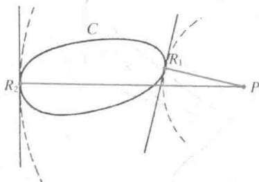
图 184 到曲线的极值距离
