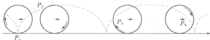
图 53 旋轮线
