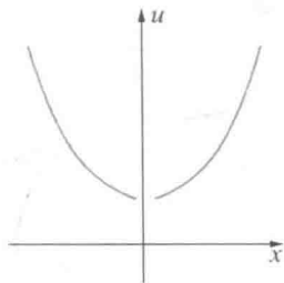
图 168 u = \frac{x + x^3}{x}
