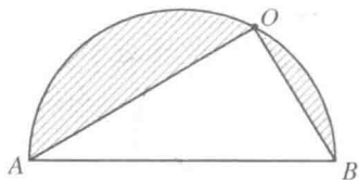
图 229
