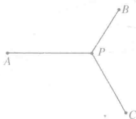
图 208 到三点的距离之和最小
