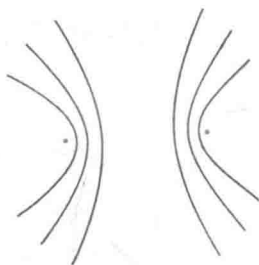
图 189 共焦点双曲线
