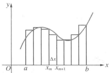
图 260 用小矩形趋近面积
