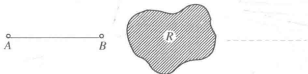
图 82 越过障碍物作一直线
