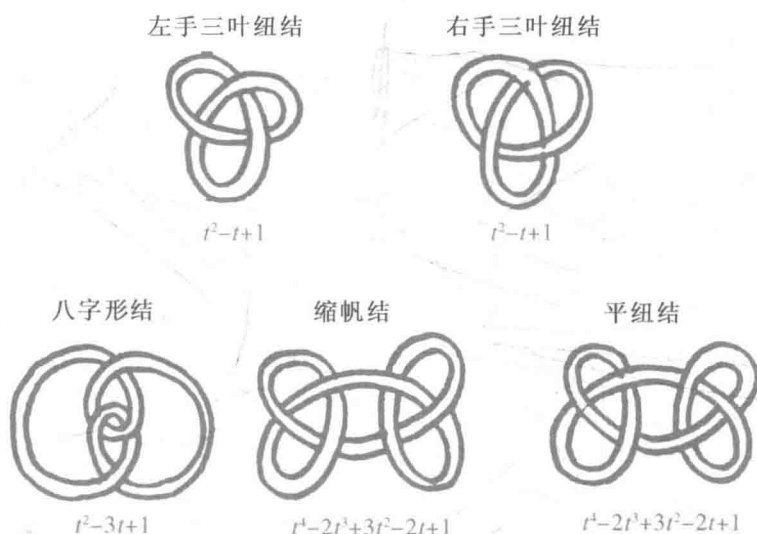
图 293 某些常见的纽结和它们的亚历山大多项式
