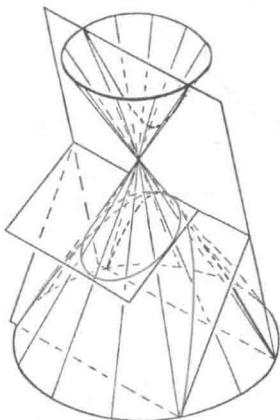
图 94 圆锥曲线
