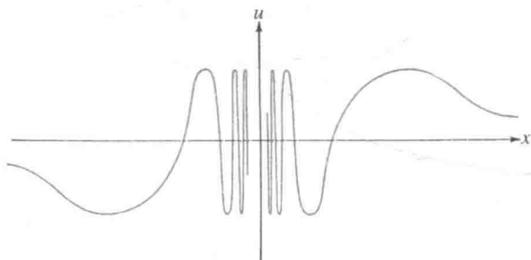
图 156 u = \sin \frac{1}{x}
