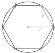
图33 正六边形
