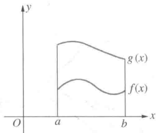
图 266 积分的比较
