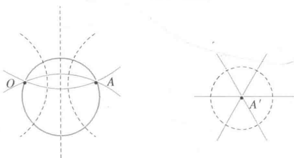
图 61 用反演相联系的两组正交圆
