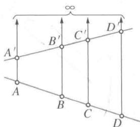
图 76 平行投影下, 交比的不变性
