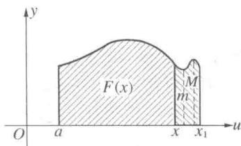
图 275 基本定理的证明
