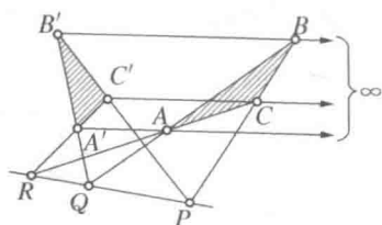
图 85 中心在无穷远处的 笛沙格图形
