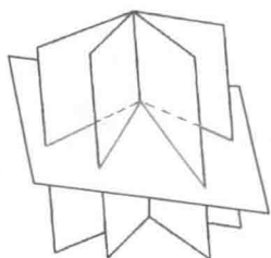
图 79 共轴平面的交比
