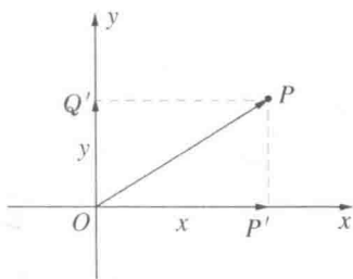
图12 一个点的直角坐标
