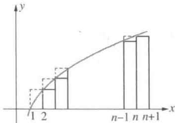
图 287 \ln(n!) 的估算
