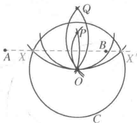
图 48 圆和不过圆心的直线的交点
