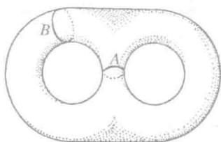
图 136 一个亏格为 2 的曲面
