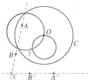
图 50 两条直线的交点
