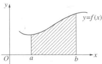
图 259 积分看作是面积
