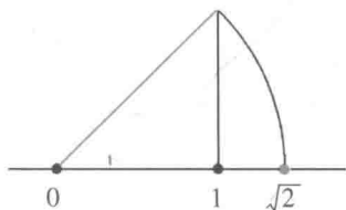
图 10 \sqrt{2} 的作图
