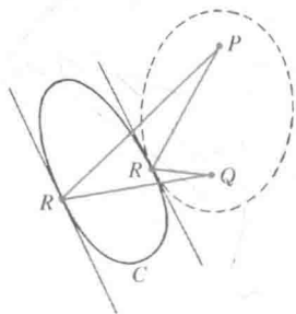
图 185 PR+QR 的最大值和最小值
