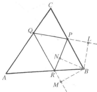
图 201
