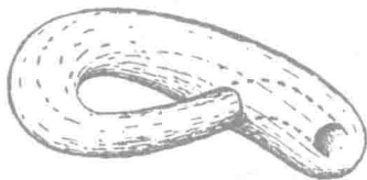
图 142 克莱茵瓶
