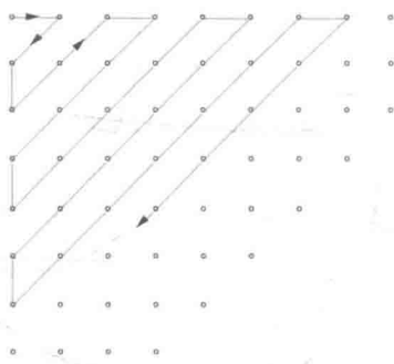
图 19 有理数的可列性
