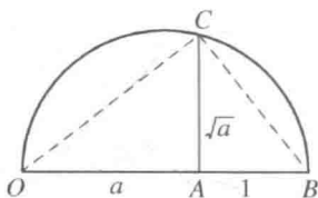
图 31 \sqrt{a} 的作图
