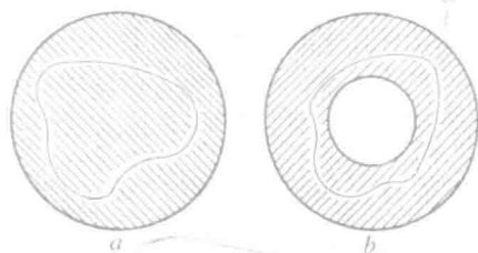
图 125 单连通和双连通
