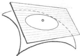
图 114 椭圆点
