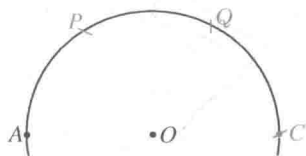
图 42 把一个线段加倍
