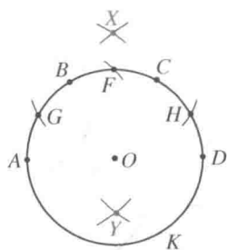
图 51 正五边形的作图
