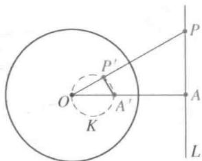
图 39 直线 L 对圆的反演
