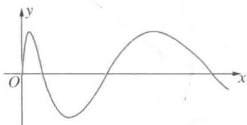
图 272 y = \sin(\sqrt{x})
