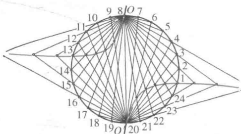
图 99 由射影产生的圆和等边双曲线
