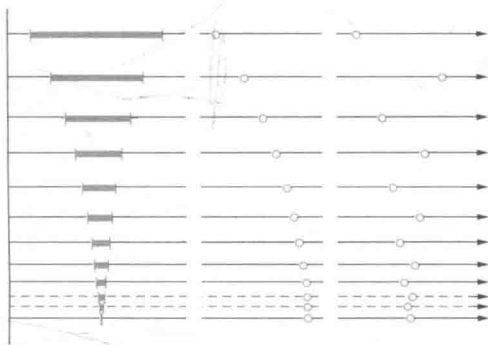
图 11 区间套 序列的极限
