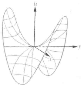
图 160 双曲抛物面
