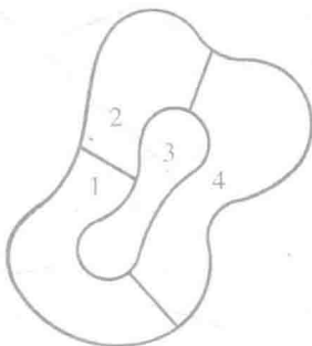
图 129 给地图上色
