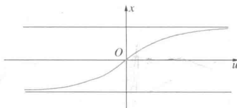
图 155 x = \arctan u
