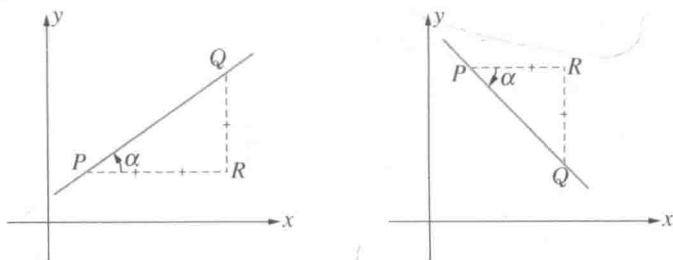
图 267 直线的斜率
