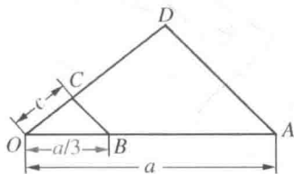
图 28 \frac{a}{3} 的作图
