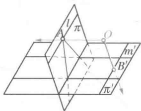
图 83 投影到无穷远
