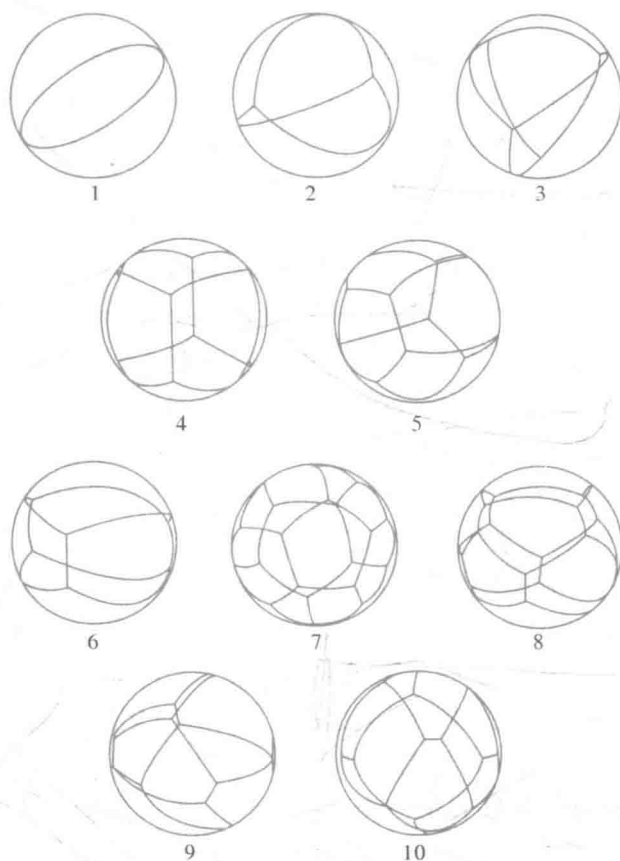
图 301 弧线交 120^\circ 的十种构形
