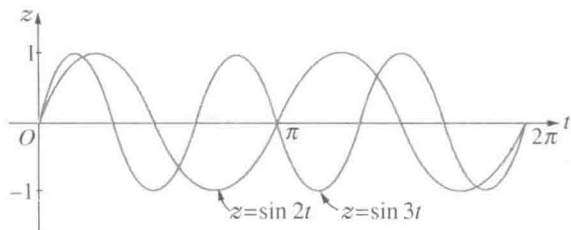
图 280
