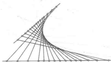
图 104 相似点类定义的抛物线
