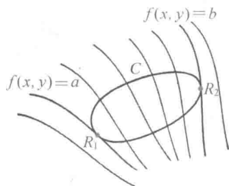
图 187 函数在曲线上的极值
