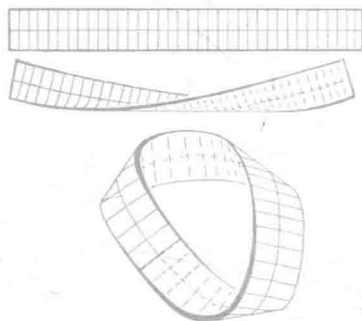
图 139 作一个莫比乌斯带
