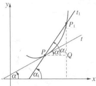
图 268 导数看作是一极限
