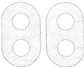
图 127 三连通区域的缩减
