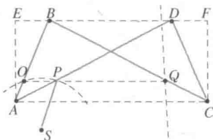
图 59 哈特的反演工具
