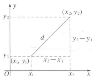
图 14 两点间距离
