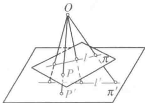
图 70 从一点投影
