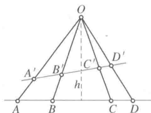
图 75 中心投影下， 交比的不变性
