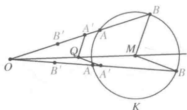
图 40 圆的反演
