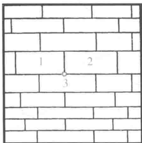
图 131 铺瓦定理
