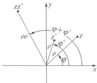
图 24 两个复数相乘, 辐角相加, 模相乘
