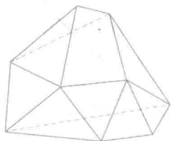
图 120 简单多面体
