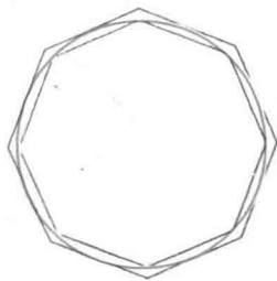
图 167 用多边形逼近圆
