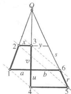
图 92 布利安桑定理的证明
