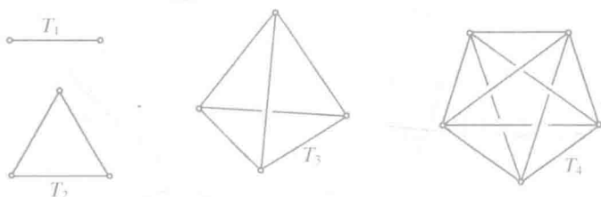
图 118 在一、二、三、四维中最简单的元素
