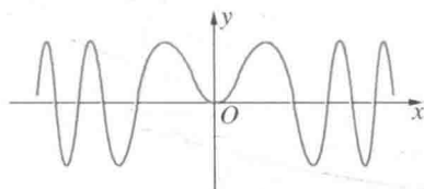
图 273 y = \sin(x^2)
