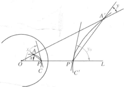
图 60 在反演下, 角的不变性
