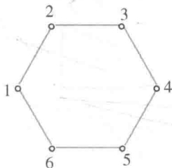
图 89
