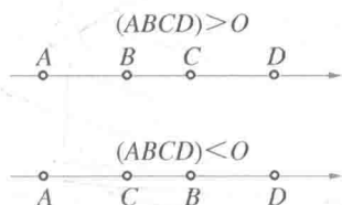
图 77 交比的符号
