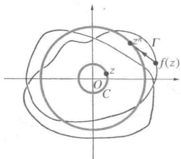
图 150 代数基本定理的证明
