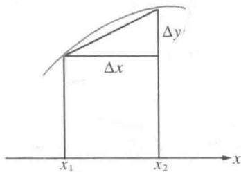
图 286 弧长
