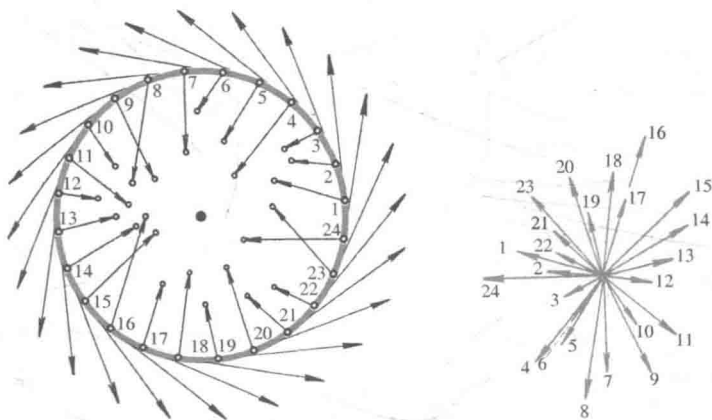
图 133
