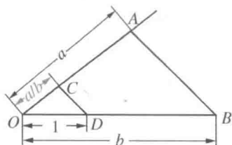
图 29 \frac{a}{b} 的作图
