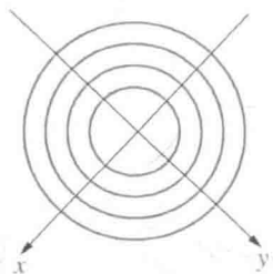
图 165 右上图中相应的等高线
