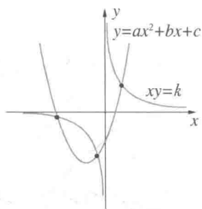
图 52 三次方程的图解
