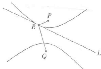
图 183 双曲线的切线性质
