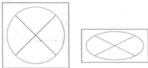
图 69 圆的压缩
