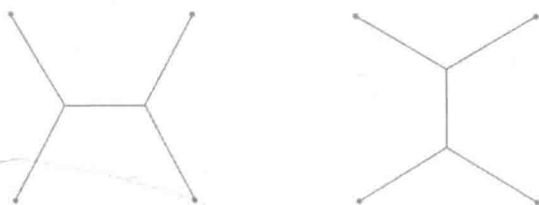
图 219~220 连接四点的两个最短网络
