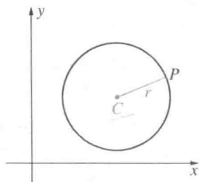
图 15 圆
