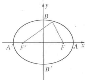
图 16 椭圆; F 和 F' 是焦点
