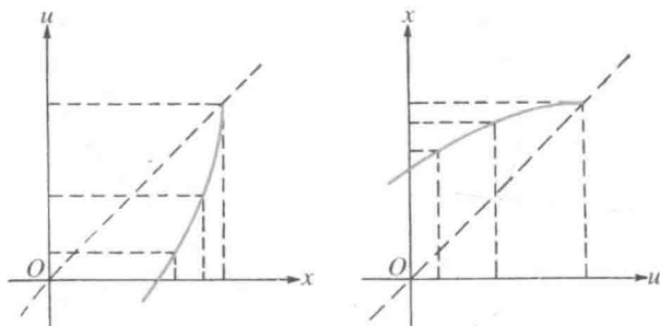
图 154 反函数
