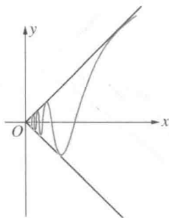
图 285 y = x \sin \frac{1}{x}
