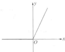
图 282 y = x + |x|
