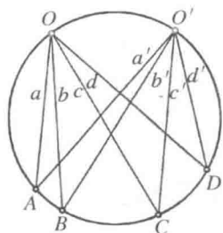
图 96 圆上的交比
