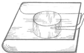
图 253 面积给定后圆有最短周长的演示
