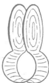
图 246
