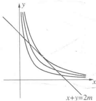
图 221 给定 x+y 时, xy 的极大值
