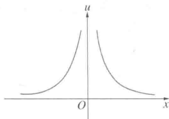
图 158 无穷的不连续
