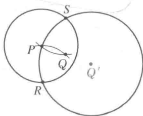
图 45 求圆心
