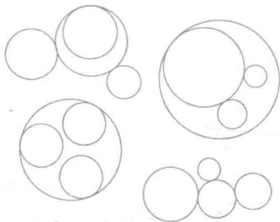
图 35 阿波罗尼斯圆
