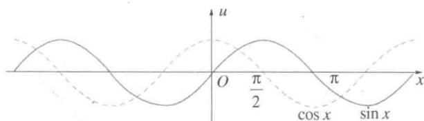
图 151 \sin x 和 \cos x 的图像
