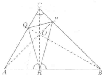
图 197 标明了等角的垂足三角形 ABC
