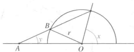
图 36 阿基米德的分角
