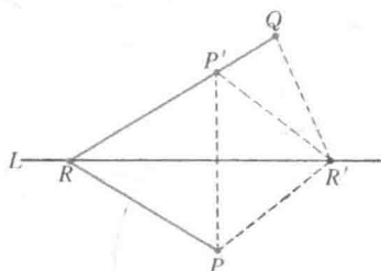
图 182 |PR - QR| = \text{极大值}
