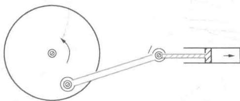
图 57 旋转转化为直线运动
