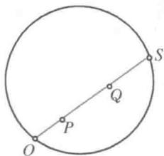
图 111 非欧几里得距离
