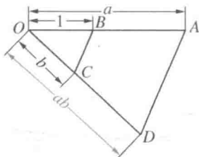
图 30 ab 的作图
