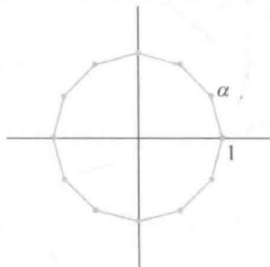
图 25 1 的 12 次方根
