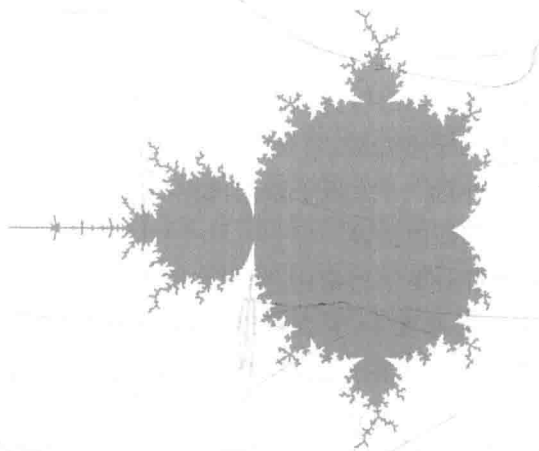
图 288 具有一切放大尺度精细结构的曼德勃罗特集
