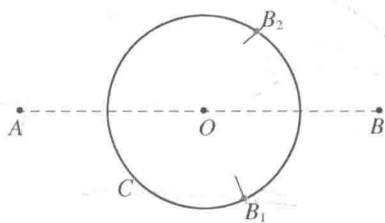
图 49 圆和过圆心的直线的交点
