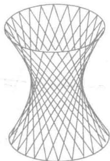
图 109 双曲面
