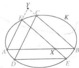
图 107 帕斯卡定理的证明
