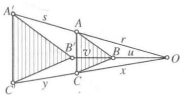
图 87 笛沙格定理的证明
