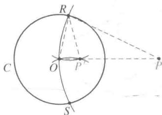
图 41 圆外一点的反演
