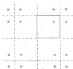
图 65 在矩形墙中的重复反射
