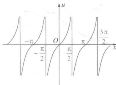
图 152 u = \tan x
