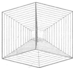
图 258
