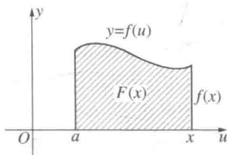
图 274 积分作为上限的函数
