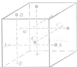
图 144 用边界的同一定义 三维曲面
