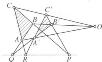
图 72 平面中笛沙格图形
