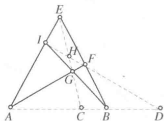
图 81 完全四边形
