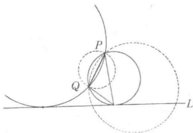
图 190 L 上使 PQ 所张的角为最大的点
