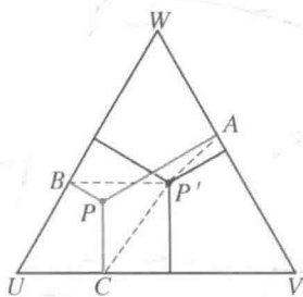
图 214 施泰纳解的另一种证法
