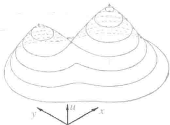
图 161 u = f(x, y) 的曲面
