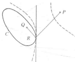
图 186 PR-QR 的最小值
