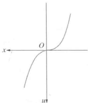
图 153 u = x^3
