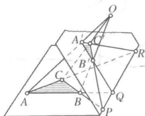
图 73 空间中笛沙格构形
