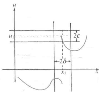
图 171 在 x = x_1 不连续的函数
