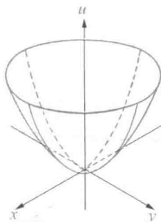
图 164 旋转抛物面
