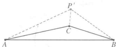
图 213 a+b+c = \text{极小值}
