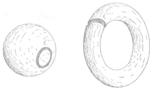
图 135 切割球和圆环
