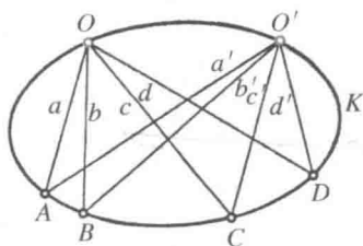
图 97 椭圆上的交比
