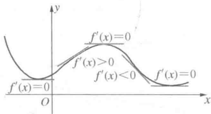
图 269 导数的符号
