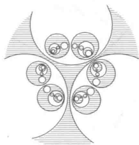
图 68 三个圆的重复反射
