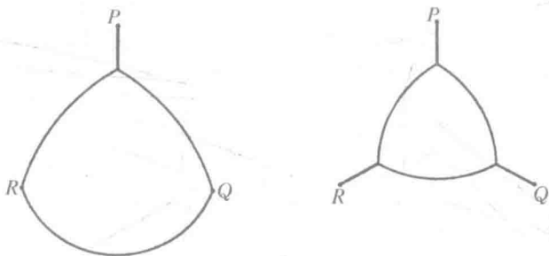
图 254~255 在一定边界条件下的等周问题
