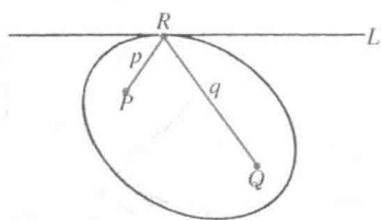
图 181 椭圆的切线性质
