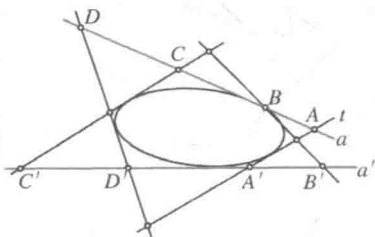
图 102 椭圆的两条切线上的射影点类
