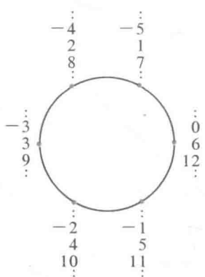
图7 模6的整数的几何表示
