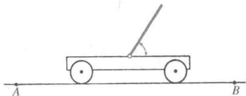
图 175
