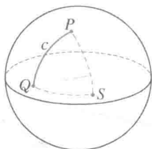
图 239 球面上的测地线
