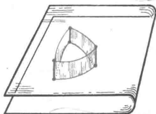
图 256
