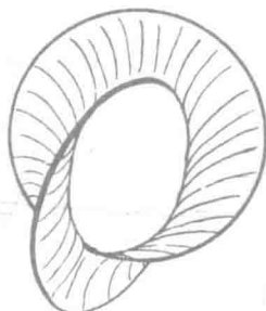
图 248 钩着的曲线
