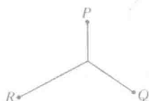
图 235
