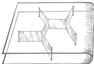
图 250 五点间的最短连线
