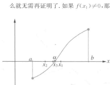
图 172 布尔查诺定理
