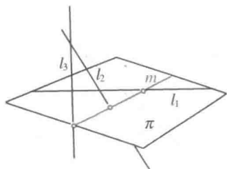
图 108 与一般位置上三条固定直线相交的直线的作图
