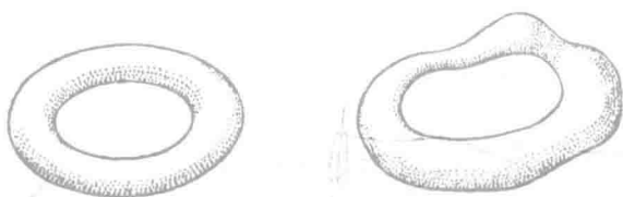
图 123 拓扑等价曲面
