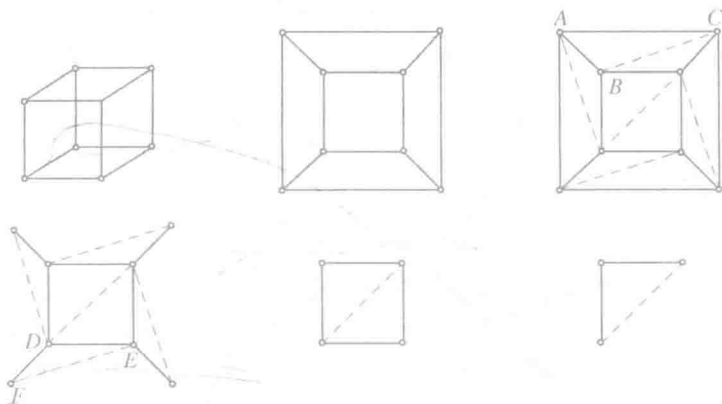
图 122 欧拉定理的证明
