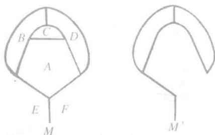
图 147
