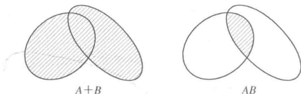
图 26 集合的并和交
