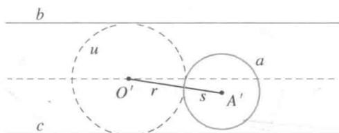
图 64 阿波罗尼斯问题的解
