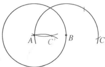
图 44 求线段中点
