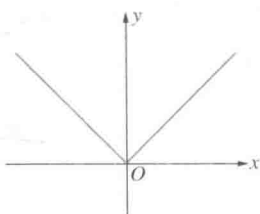
图 283 y = |x|
