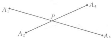
图 215 列四个点的距离之和的最小值
