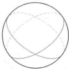
图 113 在黎曼几何中的“直线”
