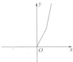
图 284 y = x + |x| + (x-1) + |x-1|
