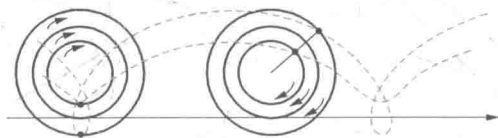
图 54 一般旋轮线
