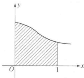
图 276 y = \frac{1}{1+x^2} 下边由 0 到 1 的面积是 \frac{\pi}{4}
