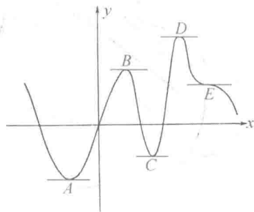
图 191 函数的驻点
