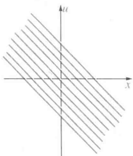
图 163 u=x+y 的等高线
