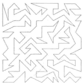
图 128 平面中哪些点是这多边形的内点?
