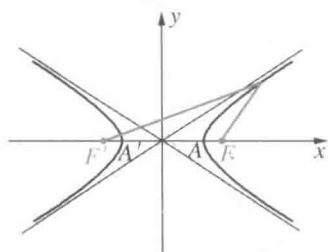
图 17 双曲线; F 和 F' 是焦点
