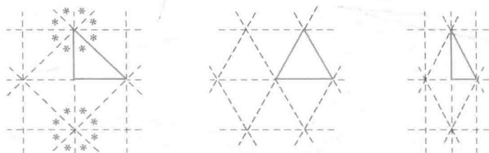
图 66 三角形镜子的规则装置
