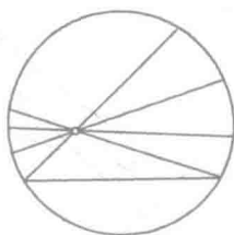
图 110 克莱茵的非欧几里得模型
