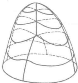
图 140 交叉帽
