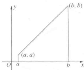
图 263 梯形的面积
