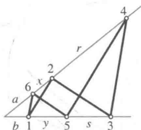
图 90 帕斯卡定理的证明
