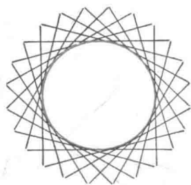
图 100 圆看作其所有切线的集合
