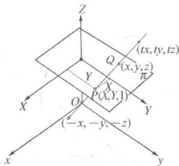
图 93 齐次坐标
