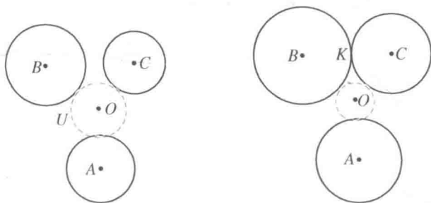
图 63 阿波罗尼斯作图的预备
