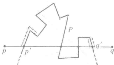
图 149
