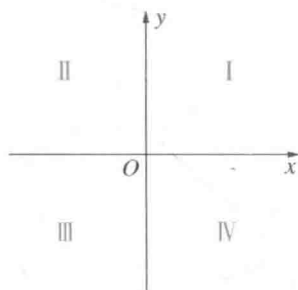
图 13 四个象限
