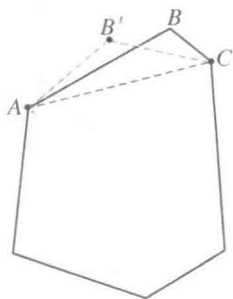
图 230
