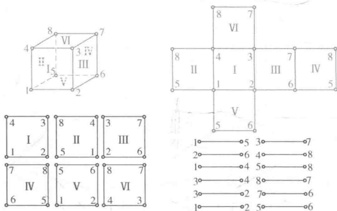
图 117 标出顶点和边来定义立方体
