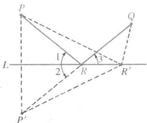
图 177 赫伦定理
