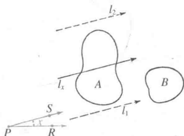
图 173 同时平分两个区域
