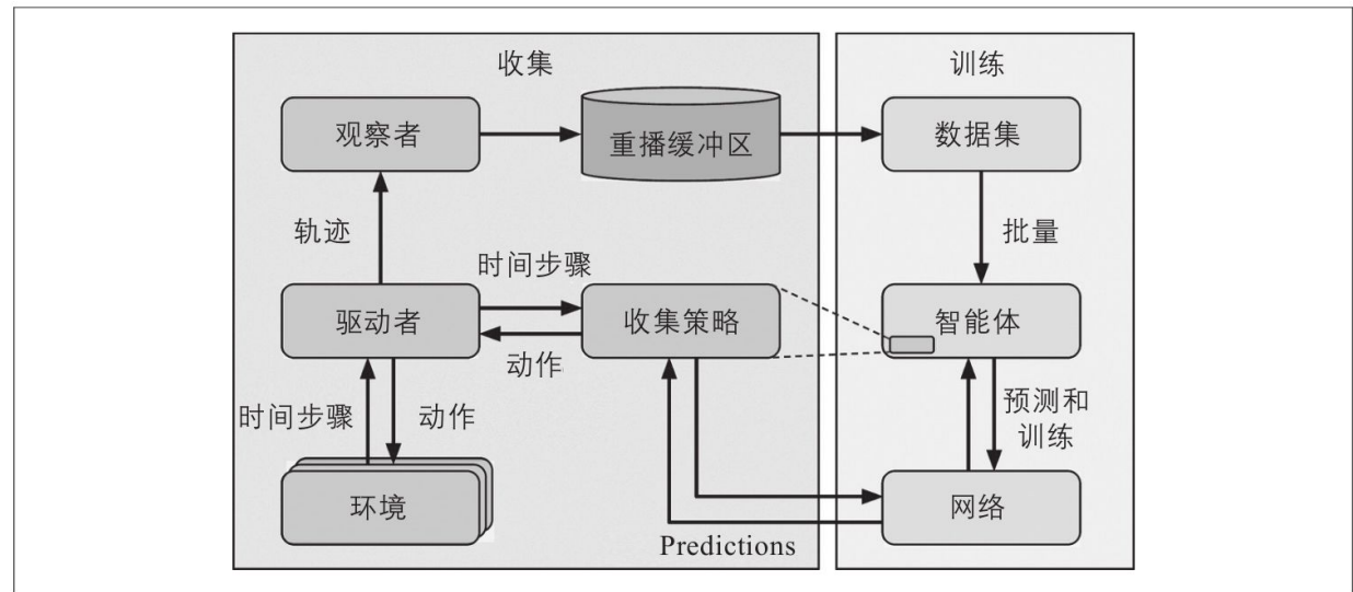
图18-13：典型的TF-Agents训练架构
