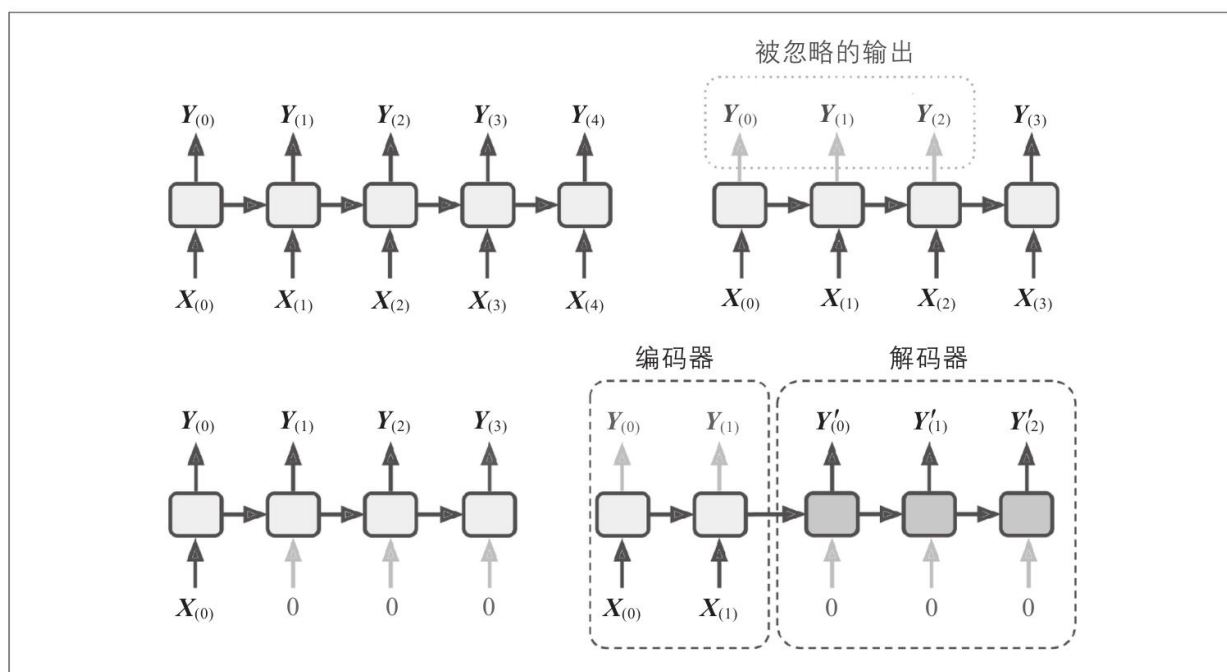
图15-4：序列到序列（左上），序列到向量（右上），向量到序列（左下）和编码器-解码器（右下）网络
