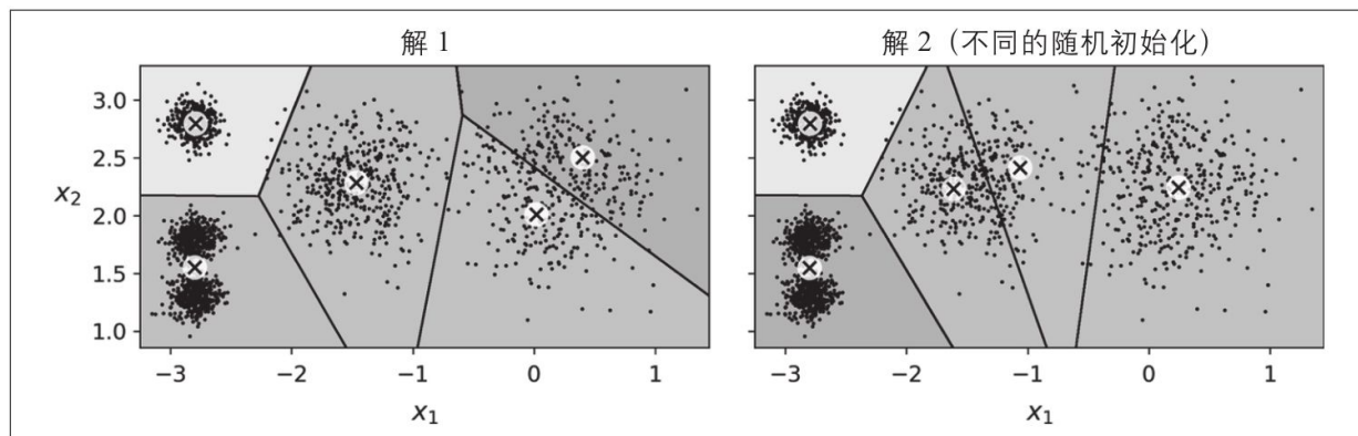
图9-5：由于中心点初始化不好而导致的次优解
