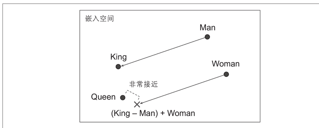
图13-5：相似词的词嵌入趋于接近，某些轴似乎编码了有意义的概念
