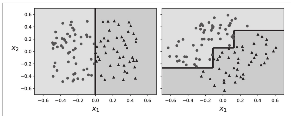
图6-7：对训练集旋转敏感
