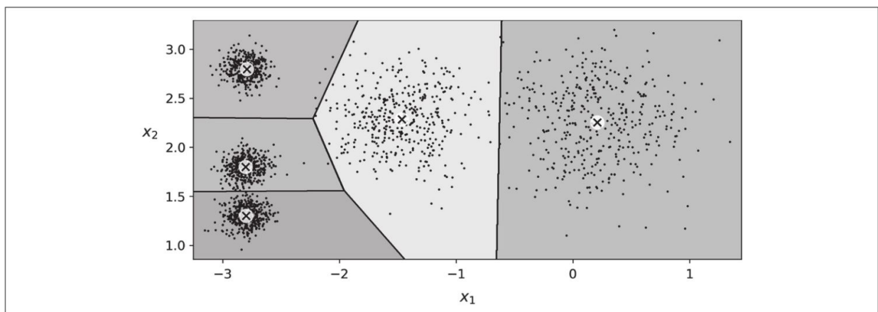
图9-3：K-Means决策边界（Voronoi图）
