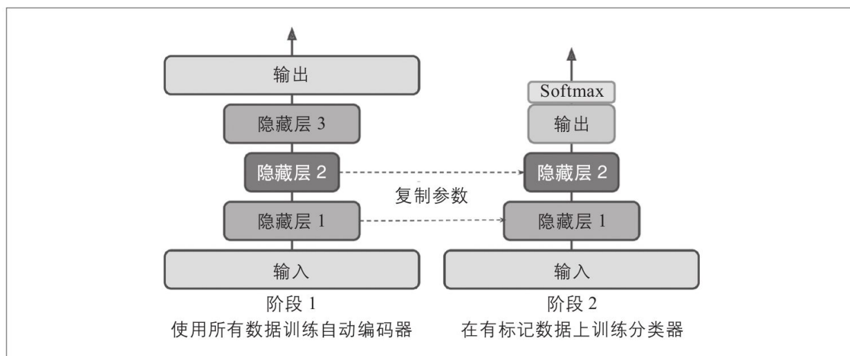
图17-6：使用自动编码器的无监督预训练
