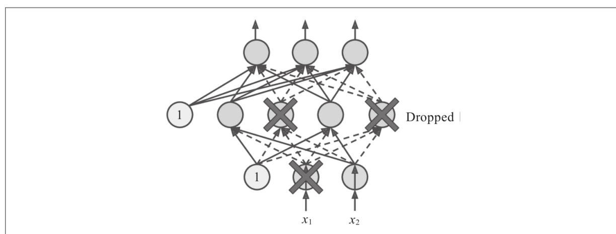
图11-9：使用dropout正则化，在每个训练迭代中，一个或多个层中的所有神经元的随机子集（输出层除外）被“删除”：这些神经元在这个迭代中输出0（用虚线箭头表示）
