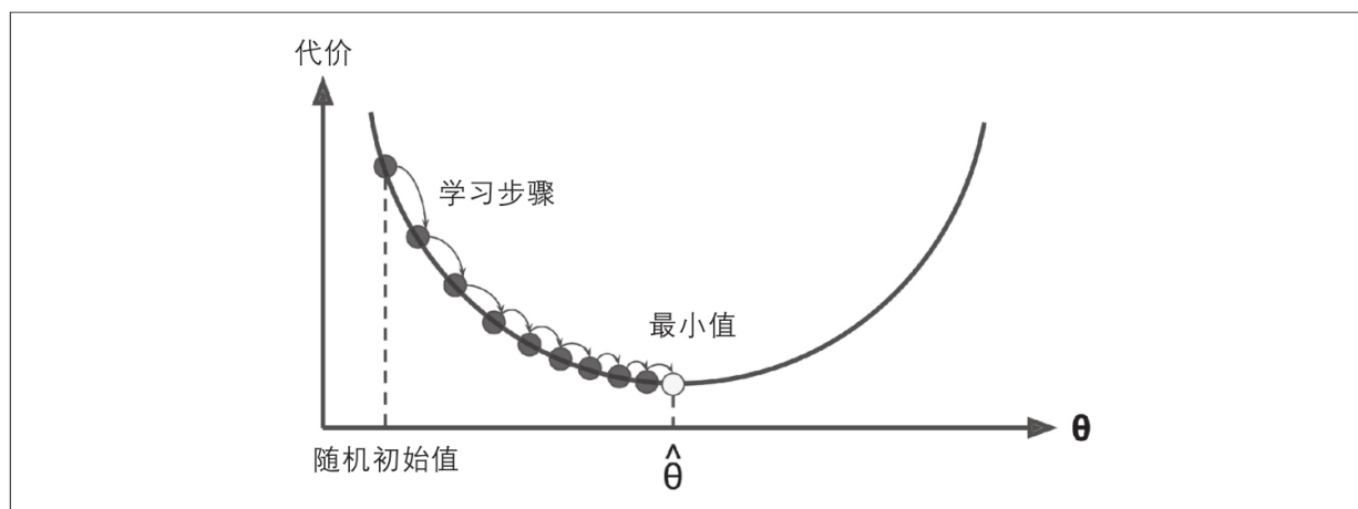
图4-3：在梯度下降的描述中，模型参数被随机初始化并反复调整使成本函数最小化。学习步长与成本函数的斜率成正比，因此，当参数接近最小值时，步长逐渐变小
