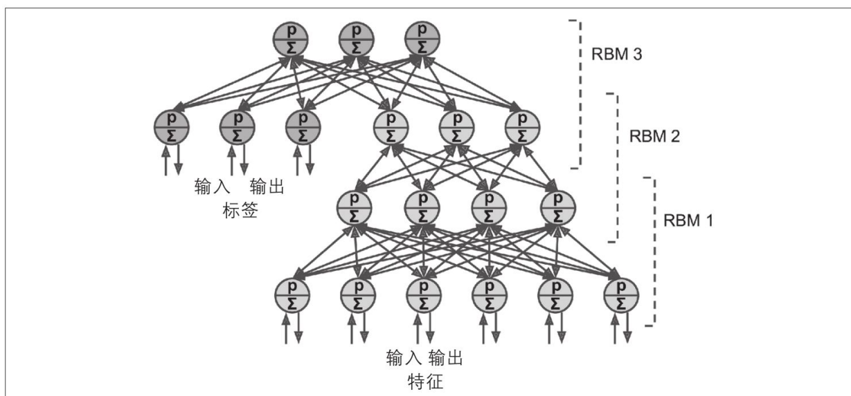
图E-4：为半监督学习配置的深度置信网络
