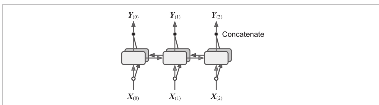
图16-5：一个双向循环层
