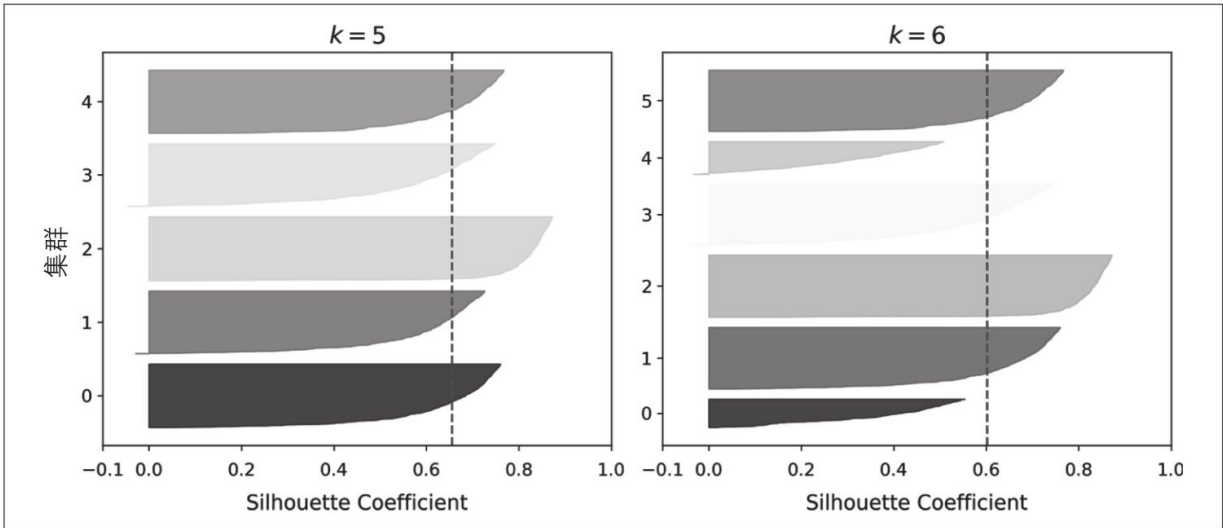
图9-10：各种K值的轮廓图分析
