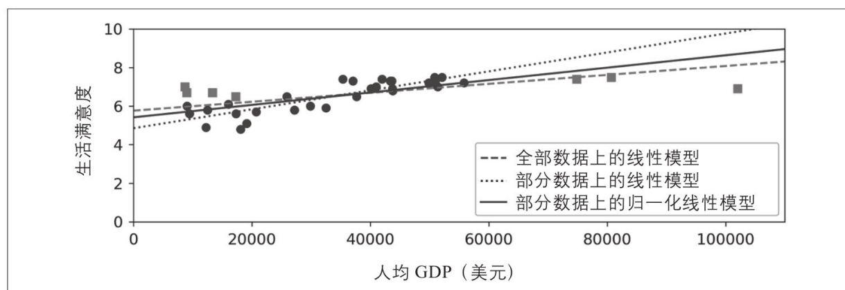
图1-23：正则化降低了过拟合的风险
