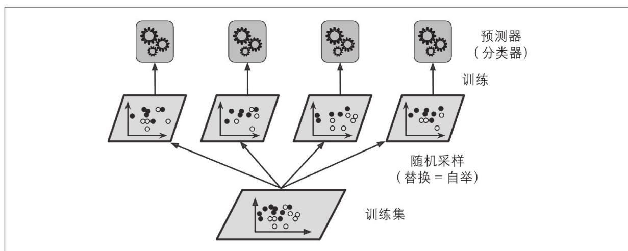
图7-4： bagging和pasting，在训练集的不同随机样本上训练几个预测器
