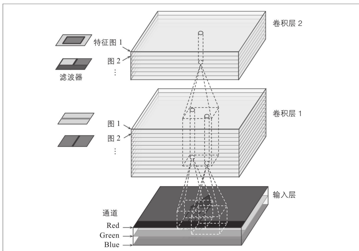
图14-6：具有多个特征图的卷积层以及具有三个颜色通道的图像
