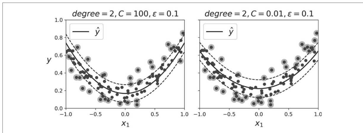
图5-11：使用二阶多项式核的SVM回归
