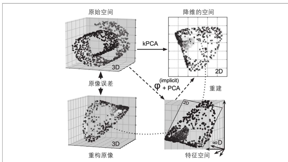
图8-11：内核PCA和重构原像误差
