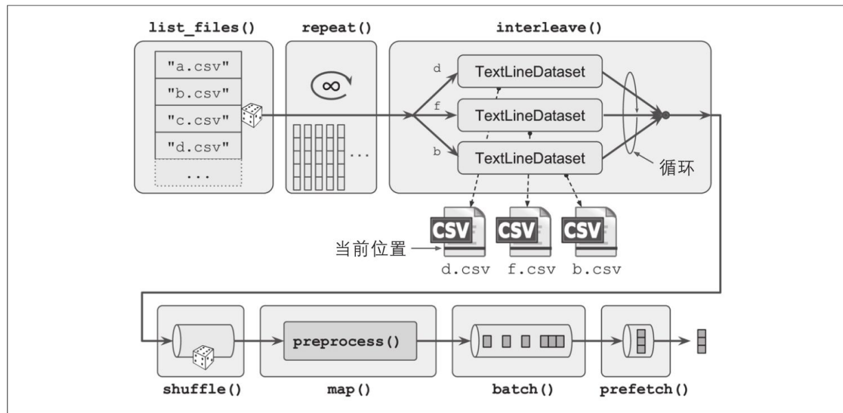
图13-2：从多个CSV文件加载和预处理数据
