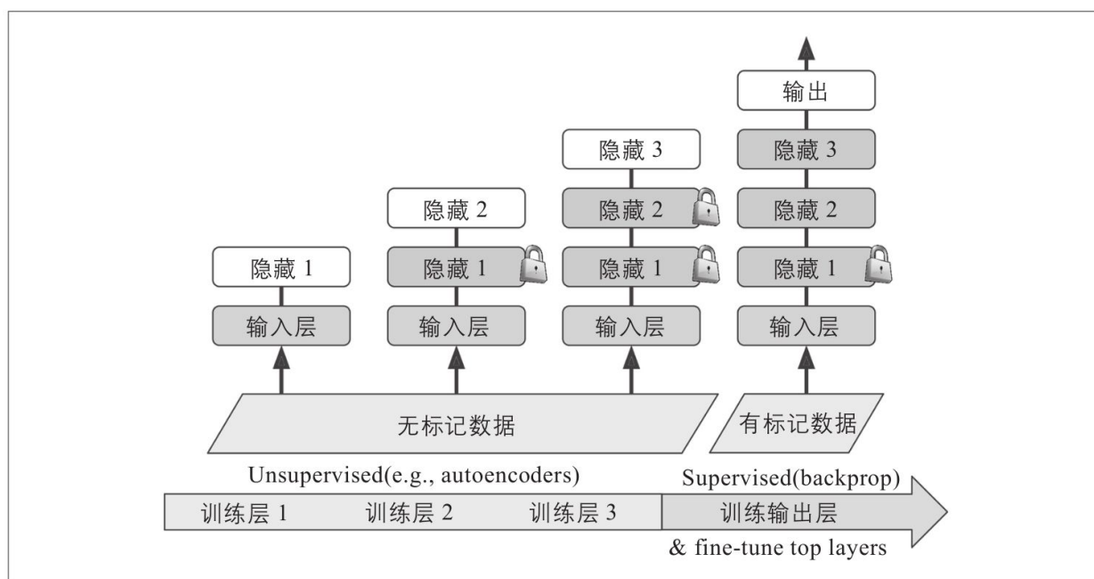
图11-5：在无监督训练中，使用一个无监督学习技术对无标记数据（或所有数据）进行训练，然后使用一个有监督学习技术对有标记数据进行最后任务的微调，无监督部分可以一次训练一层，如图所示，也可以直接训练整个模型。
