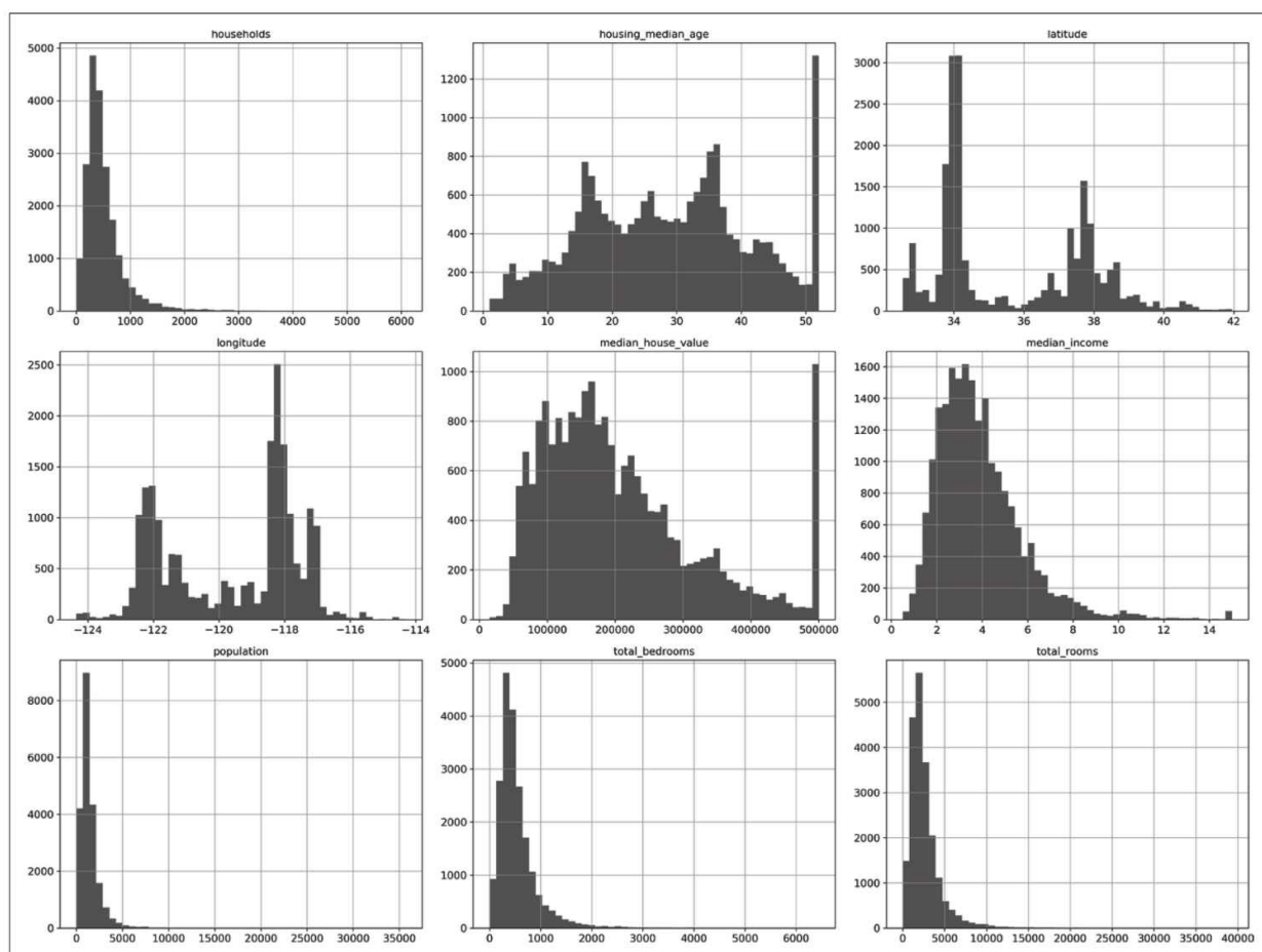
图2-8：每个数值属性的直方图
