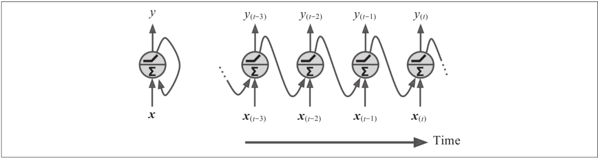
图15-1：循环神经元（左）随着时间展开（右）
