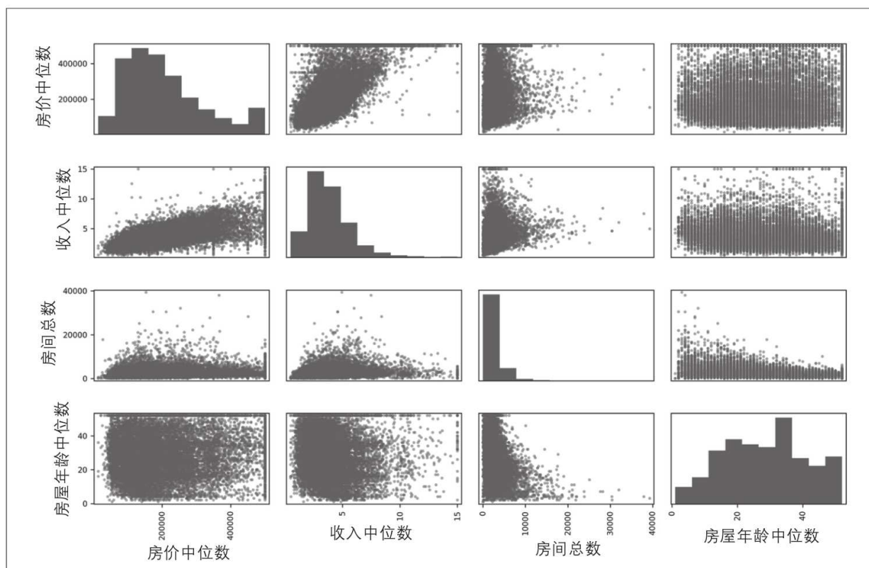
图2-15：这个散布矩阵显示每个数值属性相对于其他数值属性，并绘制每个数值属性的直方图
