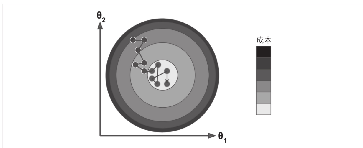
图4-9：与使用批量梯度下降相比，使用随机梯度下降时，每个训练步骤要快得多，但也更加随机
