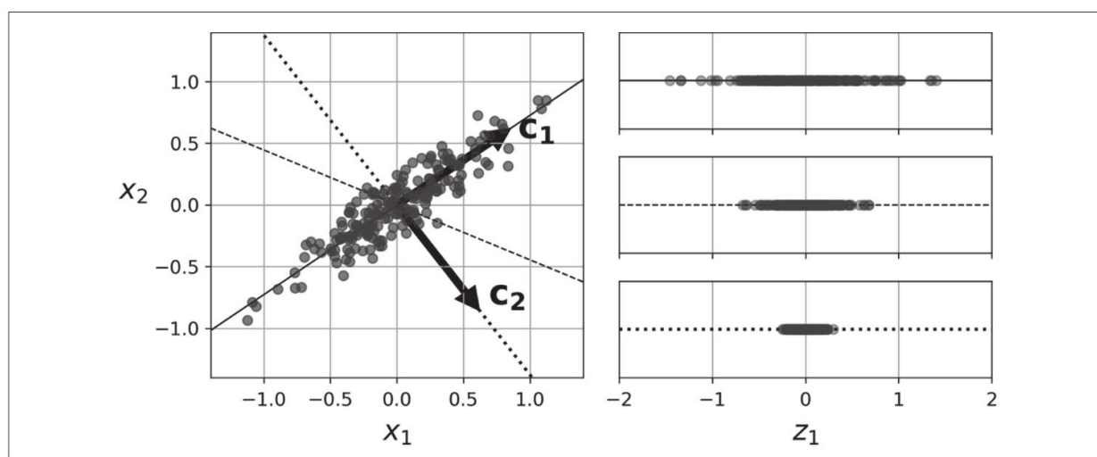
图8-7：选择要投影的子空间
