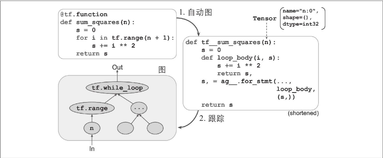
图12-4：TensorFlow如何使用自动图和跟踪生成图
