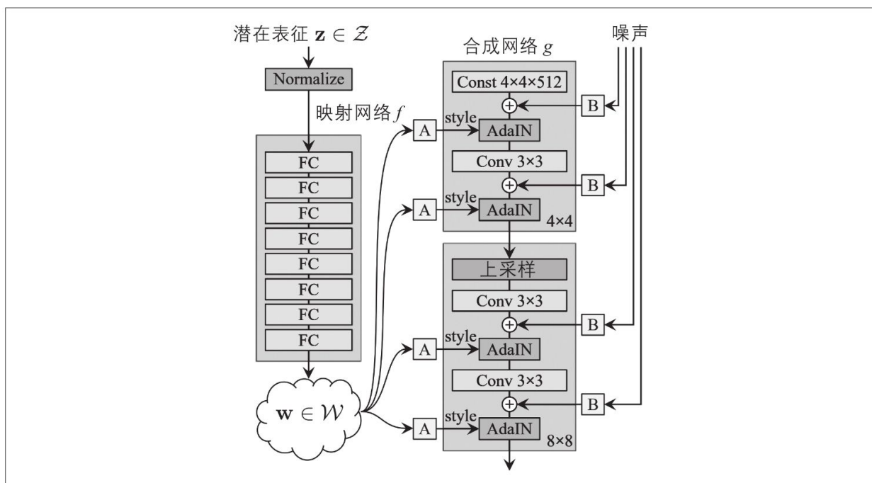
图17-20：StyleGAN的生成器架构（来自StyleGAN论文的图1的一部分） [10]
