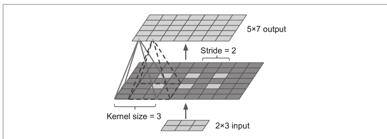
图14-27：使用转置卷积层进行上采样
