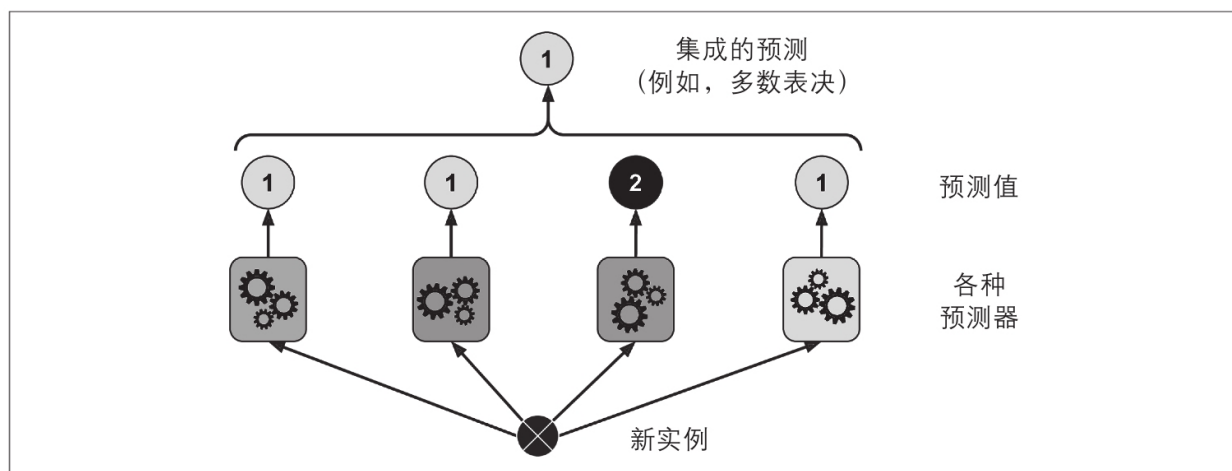
图7-2：硬投票分类器预测
