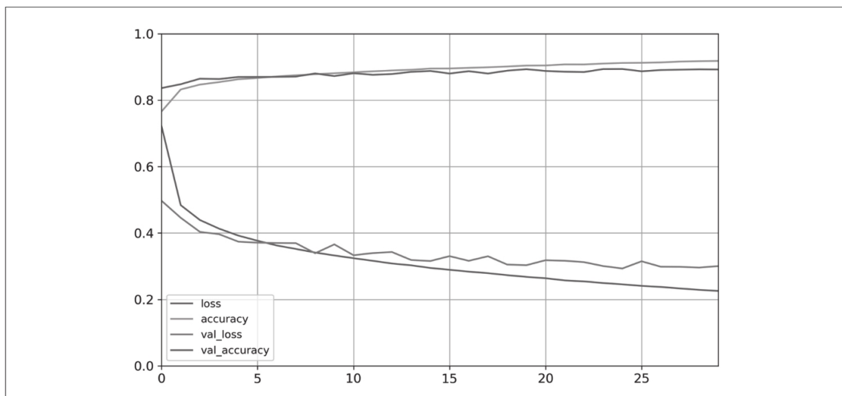
图10-12：学习曲线：每个轮次测得的平均训练损失和准确率，以及每个轮次结束时测得的平均验证损失和准确率
