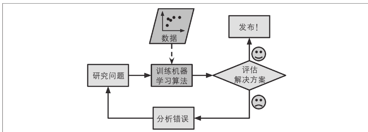
图1-2：机器学习方法
