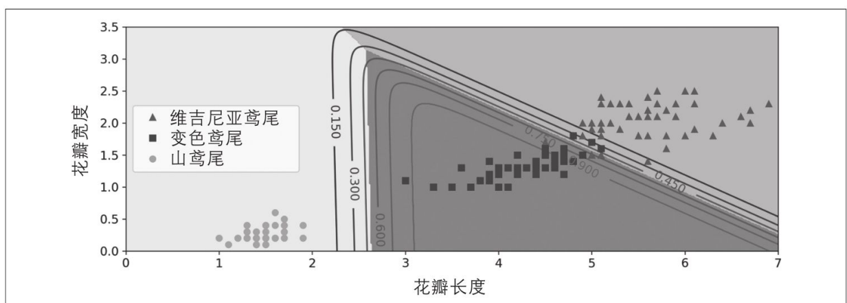
图4-25：Softmax回归决策边界
