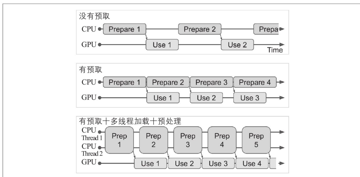
图13-3：通过预取，CPU和GPU并行工作：当GPU处理一个批次时，CPU处理下一批次
