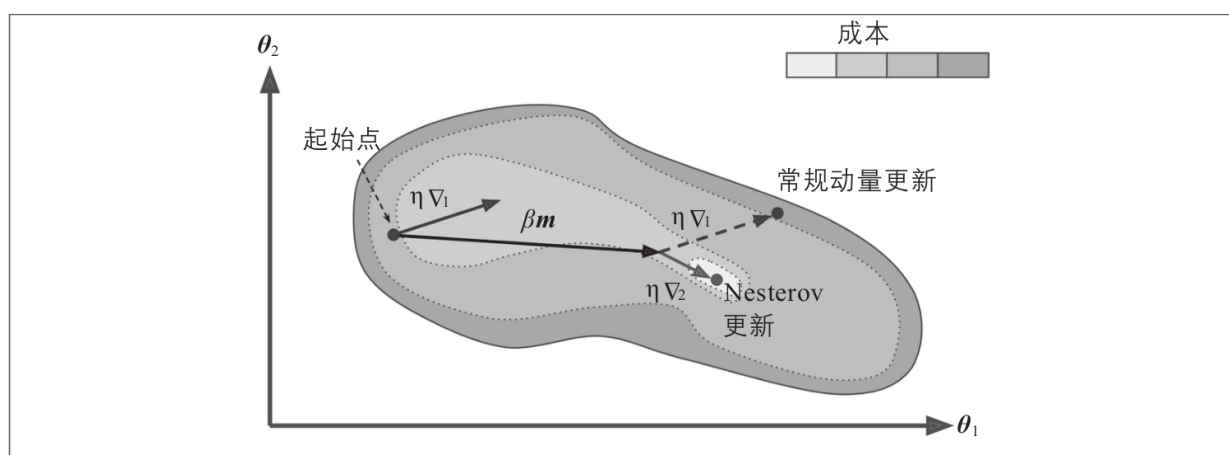
图11-6：常规与Nesterov动量优化：前者使用在动量步骤之前计算的梯度，而后者使用在动量步骤之后计算的梯度
