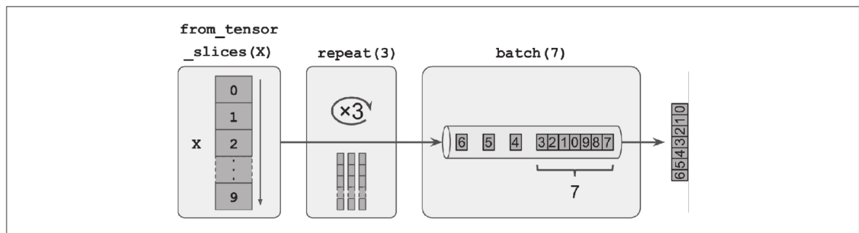
图13-1：链式数据集转换
