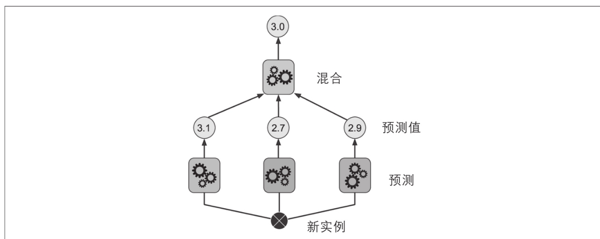
图7-12：通过混合预测器聚合预测
