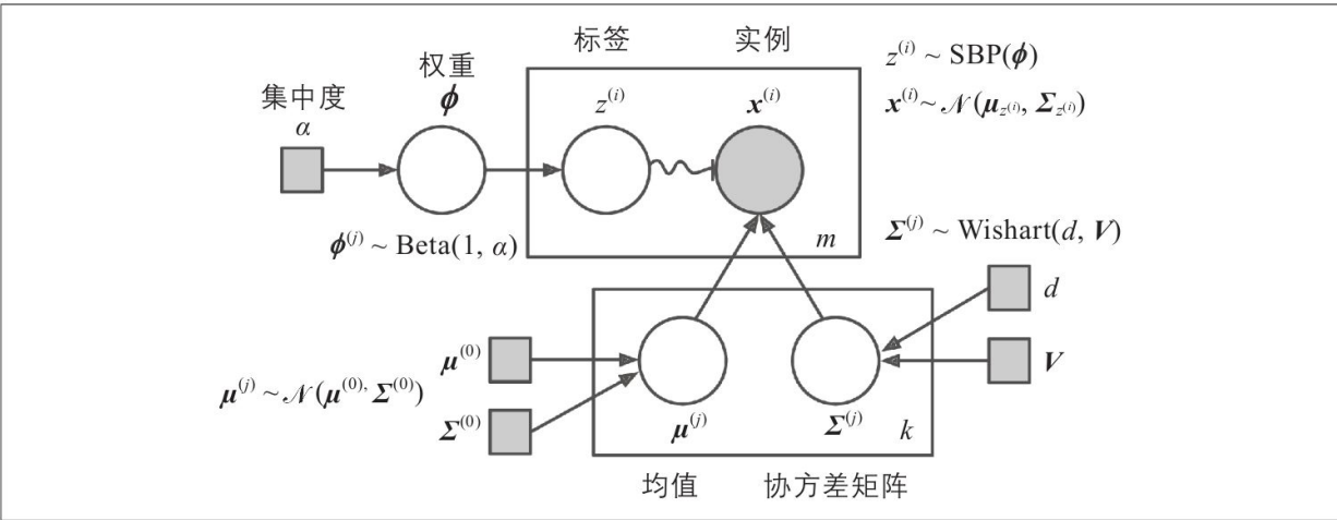
图9-22：贝叶斯高斯混合模型
