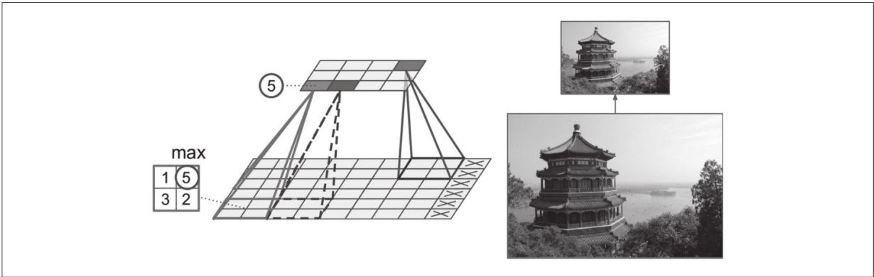
图14-8：最大池化层（ 2 \times 2 池化内核，步幅为2，无填充）
