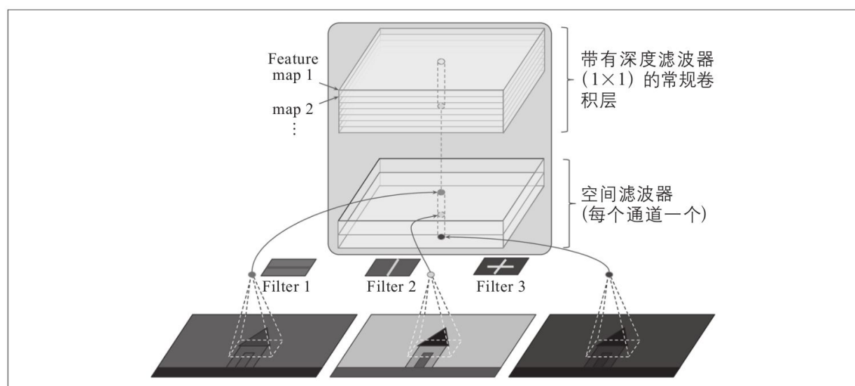
图14-19：深度可分离卷积层
