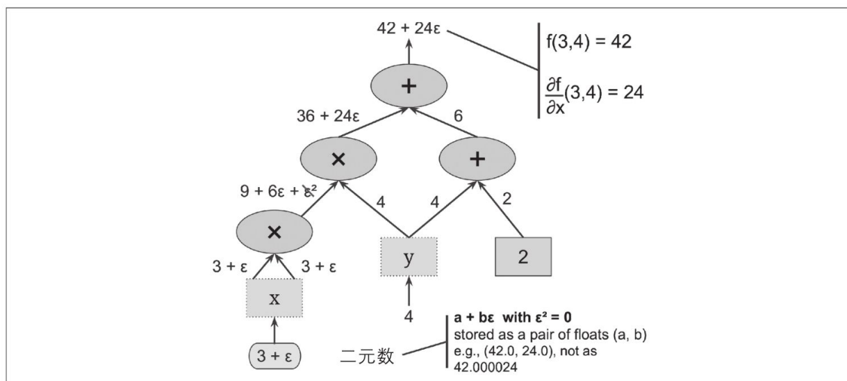
图D-2：使用二元数的前向模式自动微分
