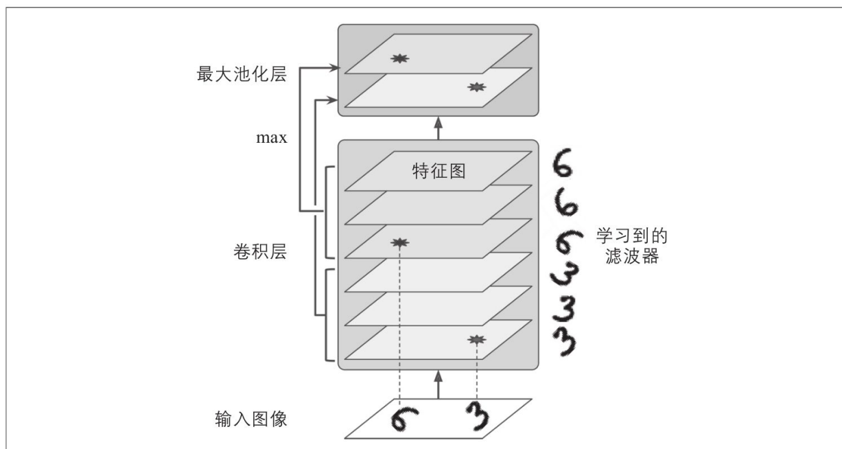
图14-10：深度最大池化可以帮助CNN学习任何不变性
