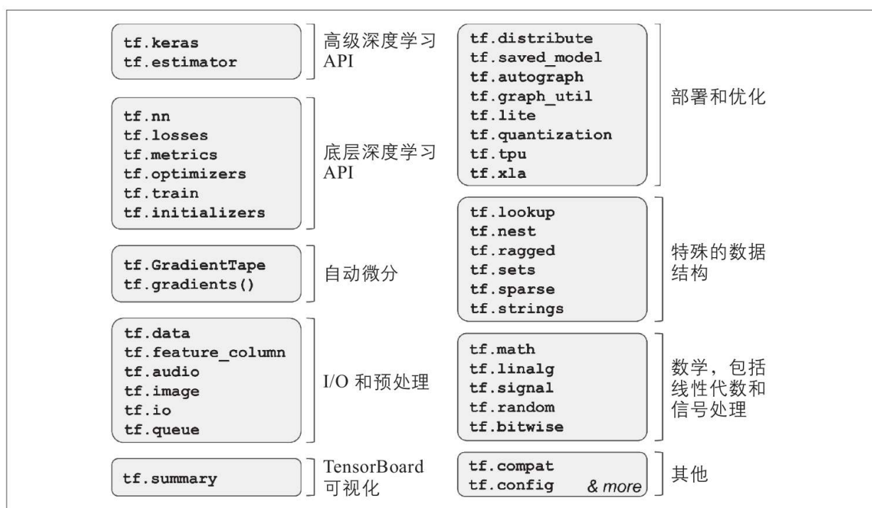
图12-1：TensorFlow的Python API
