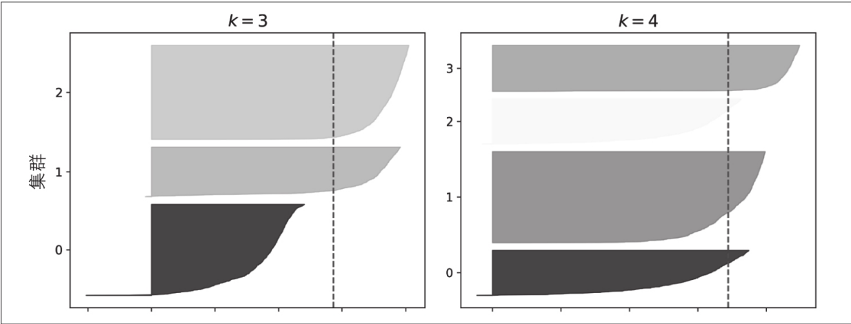
图9-10：各种K值的轮廓图分析
