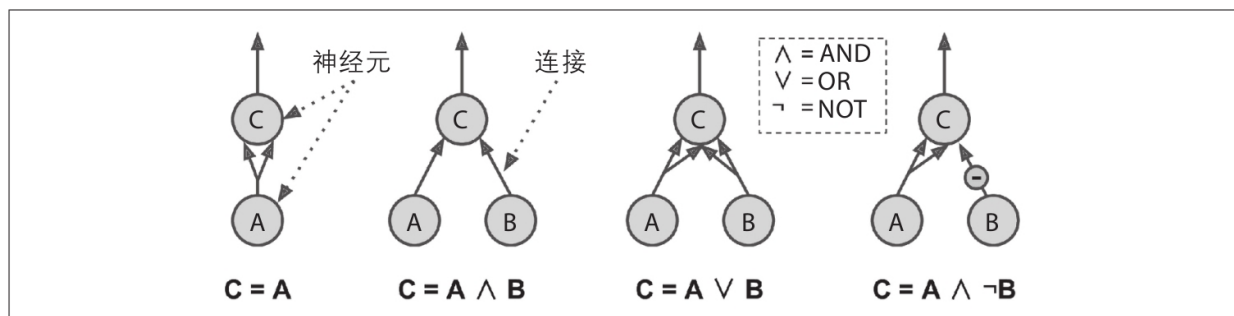
图10-3：ANN执行简单的逻辑运算
