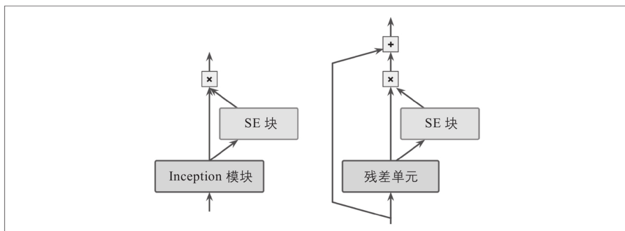
图14-20：SE-Inception模块（左）和SE-ResNet单元（右）
