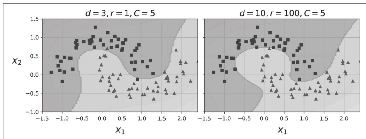
图5-7：多项式核的SVM分类器
