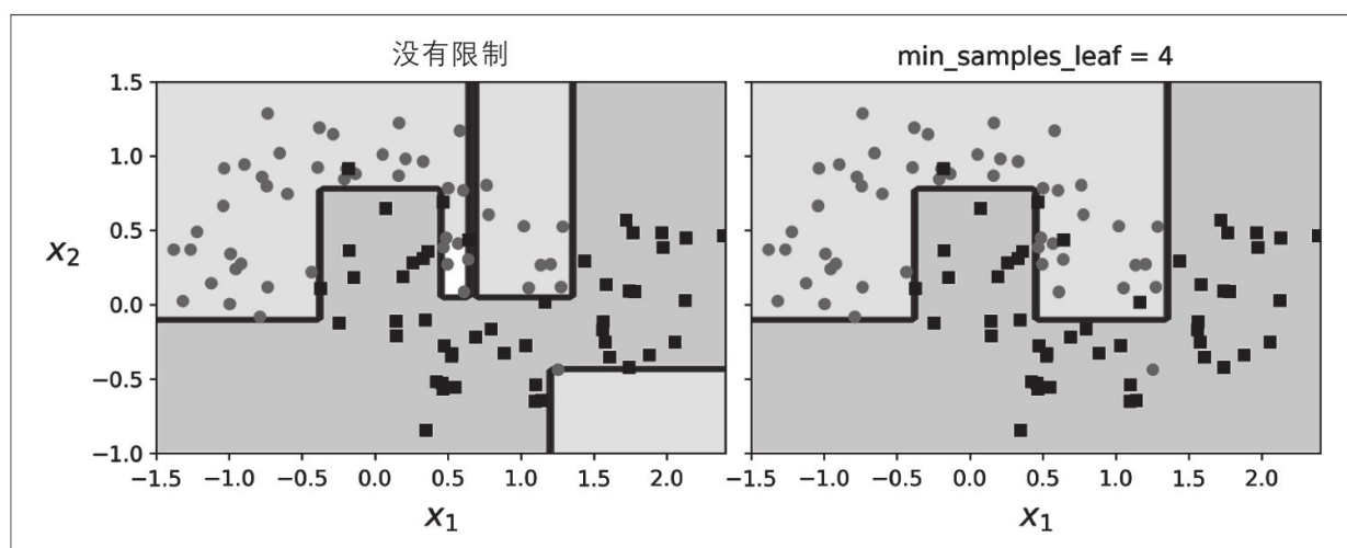
图6-3：使用 min_samples_leaf 进行正则化
