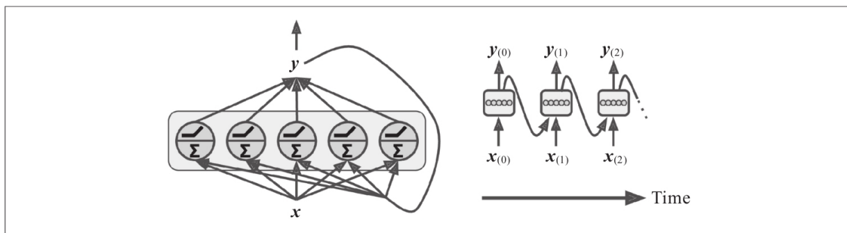
图15-2：一层循环神经元（左）随着时间展开（右）
