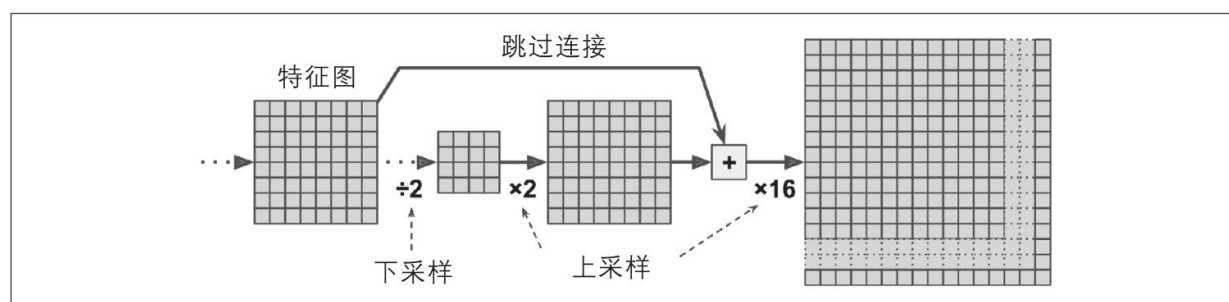
图14-28：跳过层从较低层恢复一些空间分辨率
