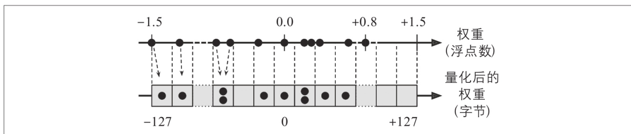
图19-8：使用对称量化，从32位浮点数到8位整数
