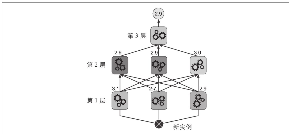
图7-15：一个多层堆叠集成的预测
