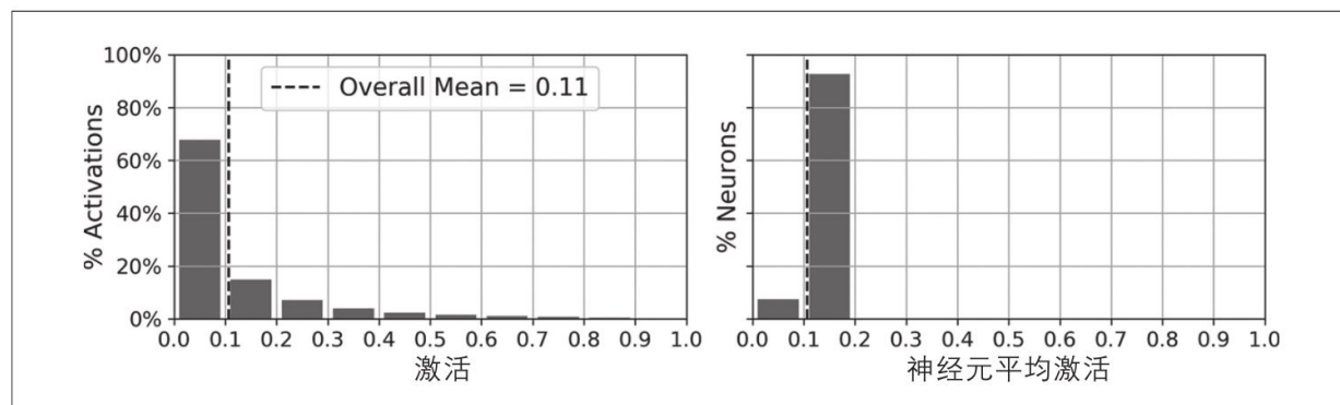
图17-11：编码层中所有激活的分布（左）和每个神经元的平均激活分布（右）
