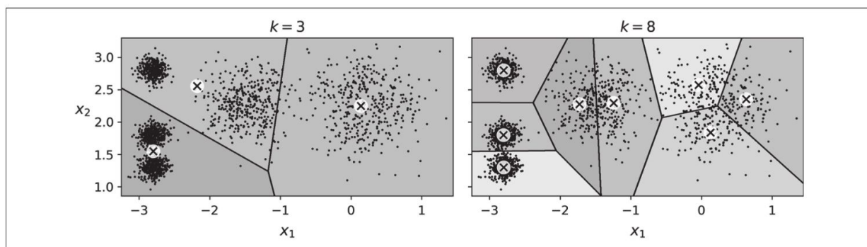
图9-7：集群数量的错误选择：当 k 太小时，单独的集群会合并（左），而当 k 太大时，某些集群会被分成多个（右）
