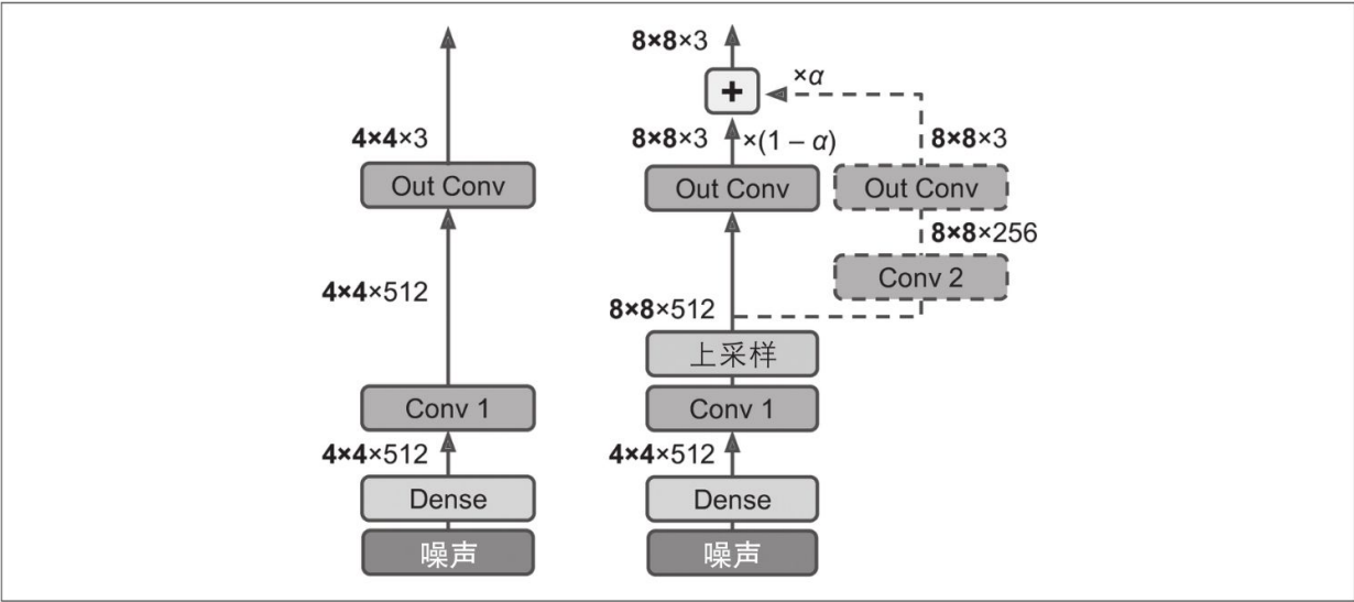
图17-19：渐进式GAN：GAN生成器输出4×4彩色图像（左）。我们扩展它以输出8×8图像（右）
