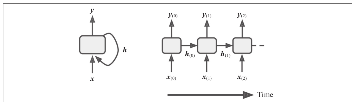
图15-3：单元的隐藏状态和其输出可能不同
