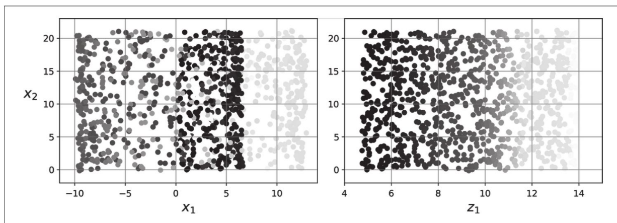
图8-5：投影到平面上（左）与展开瑞士卷（右）
