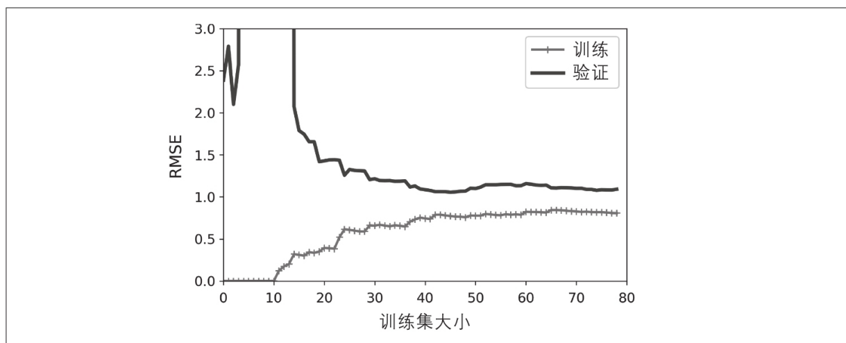
图4-16：10阶多项式模型的学习曲线
