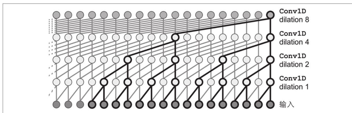
图15-11: WaveNet架构
