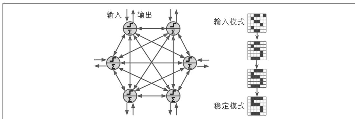
图E-1：Hopfield网络
