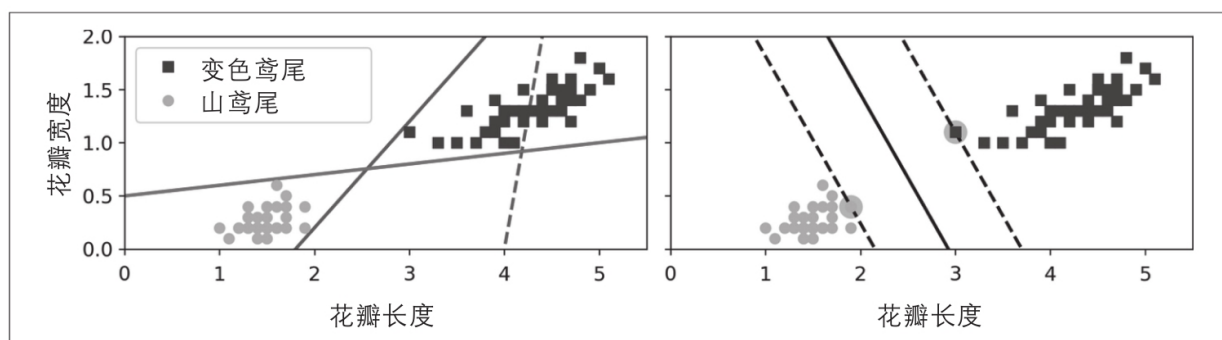
图5-1：大间隔分类
