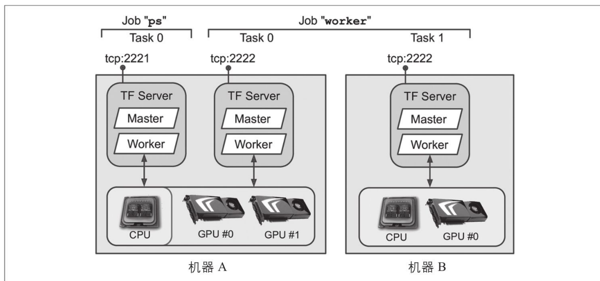
图19-21: TensorFlow集群
