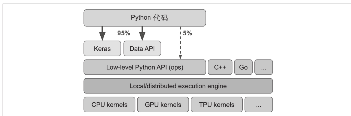
图12-2：TensorFlow的架构
