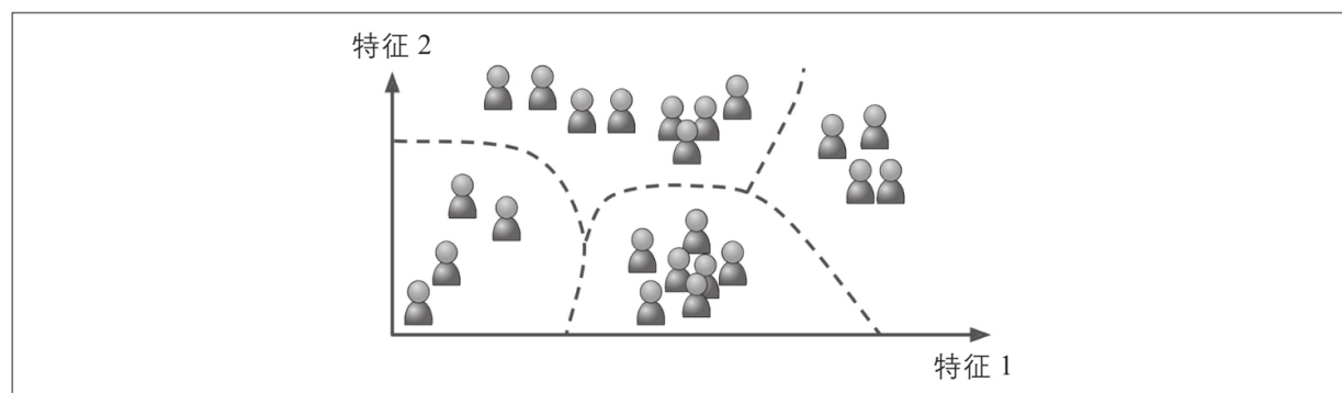
图1-8：聚类
