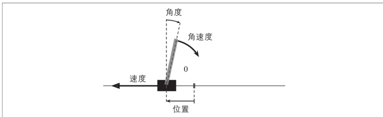
图18-4: CartPole环境
