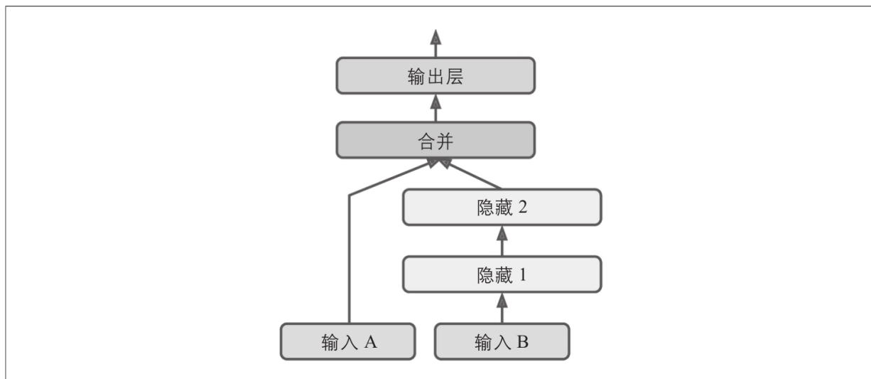
图10-15：处理多输入
