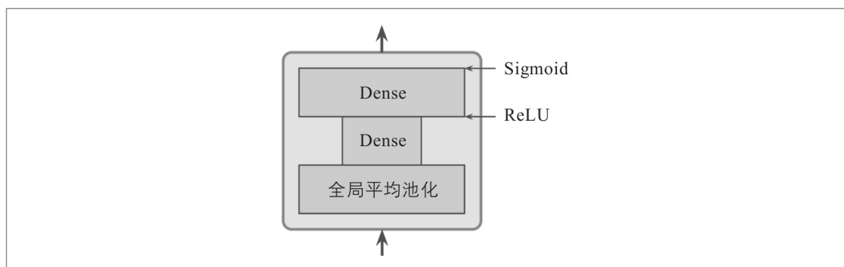
图14-22：SE块架构
