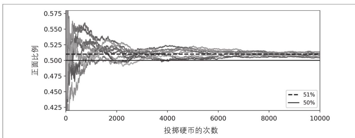
图7-3：大数定理
