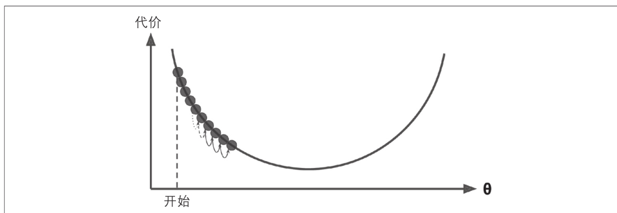
图4-4：学习率太小
