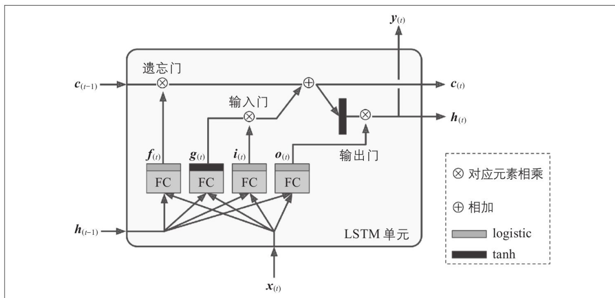
图15-9：LSTM单元
