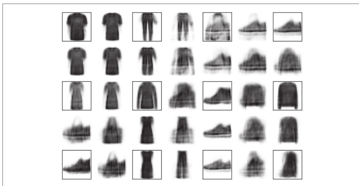
图17-14：语义插值
