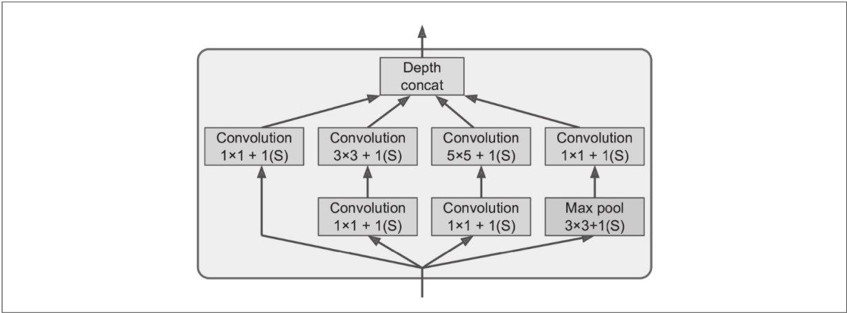
图14-13: Inception模块
