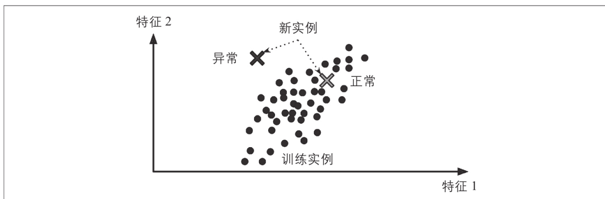
图1-10：异常检测
