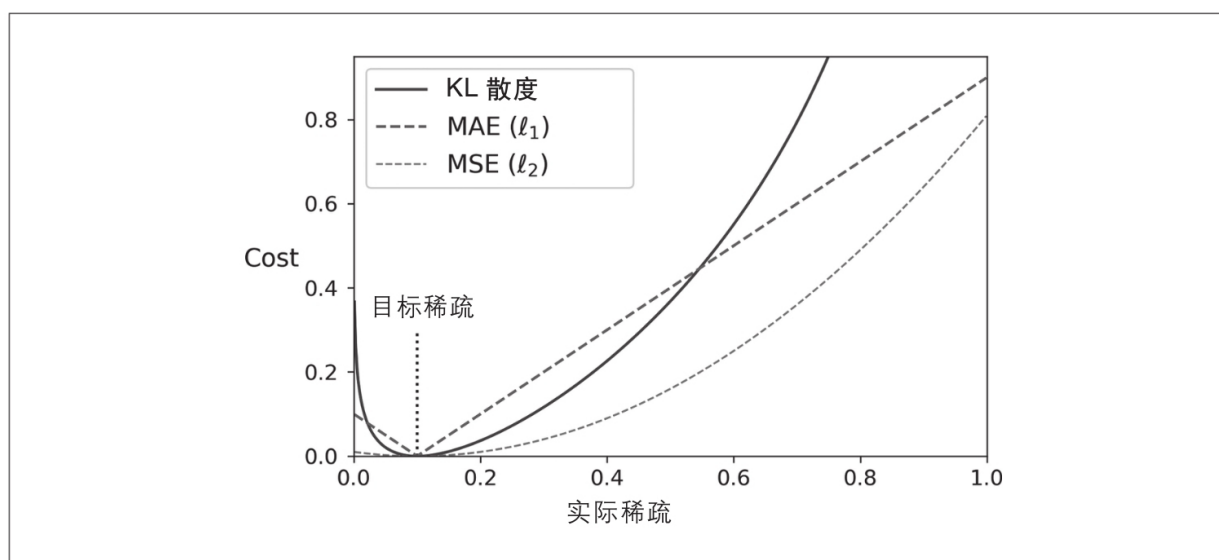
图17-10：稀疏损失
