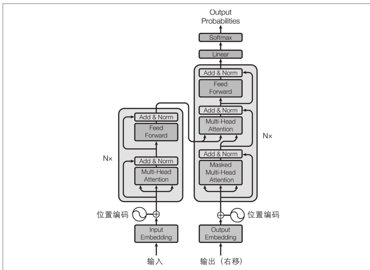
图16-8: Transformer架构 [10]
