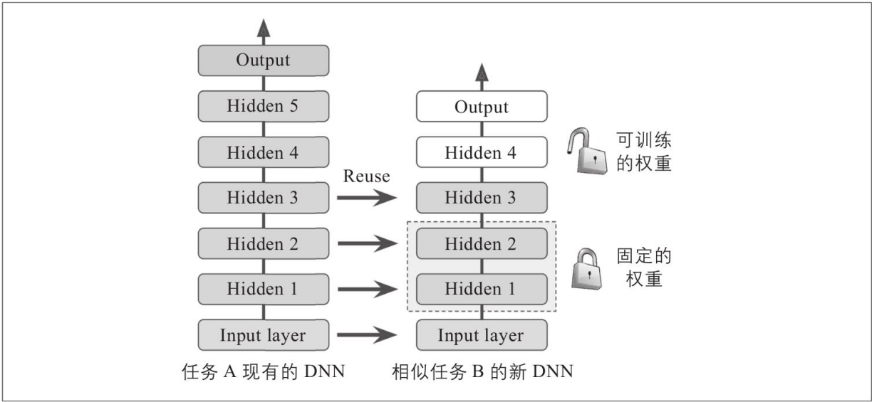
图11-4：重用预训练层
