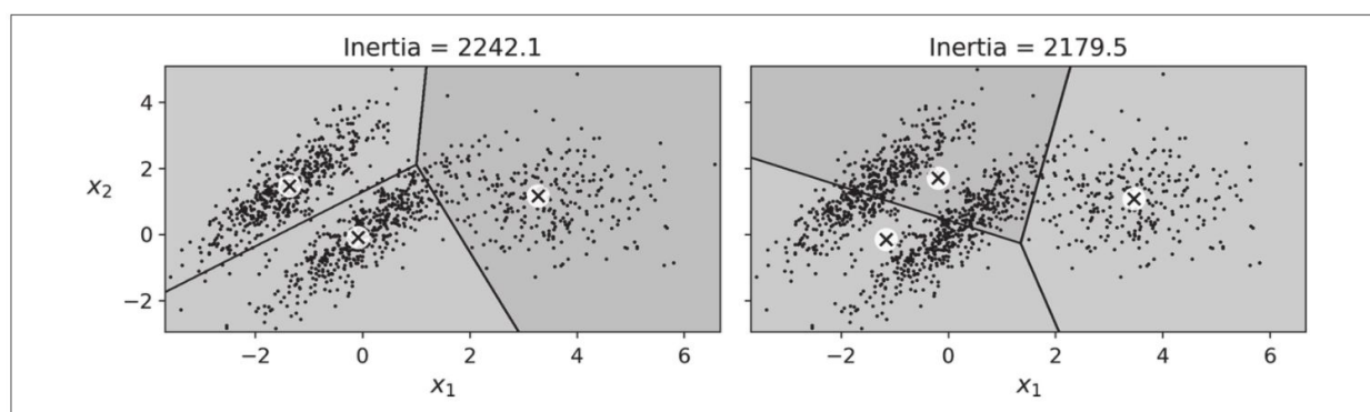
图9-11：K-Means无法正确聚类这些椭圆形集群
