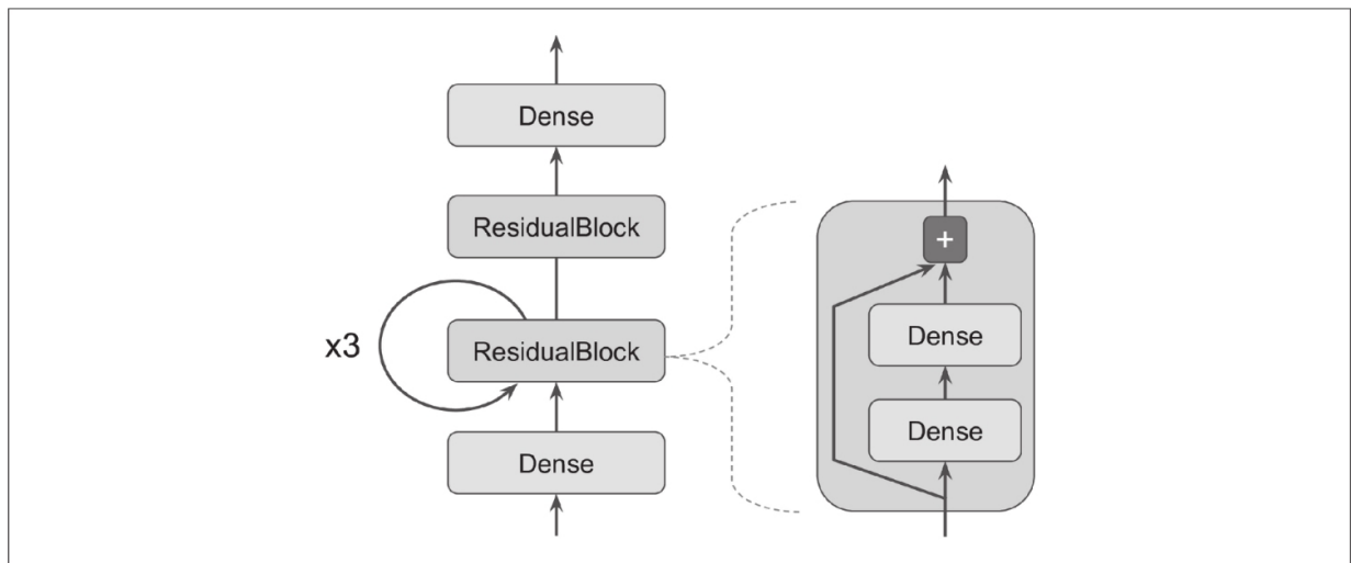
图12-3：自定义模型示例：具有自定义ResidualBlock层（包含跳过连接）的任意模型
