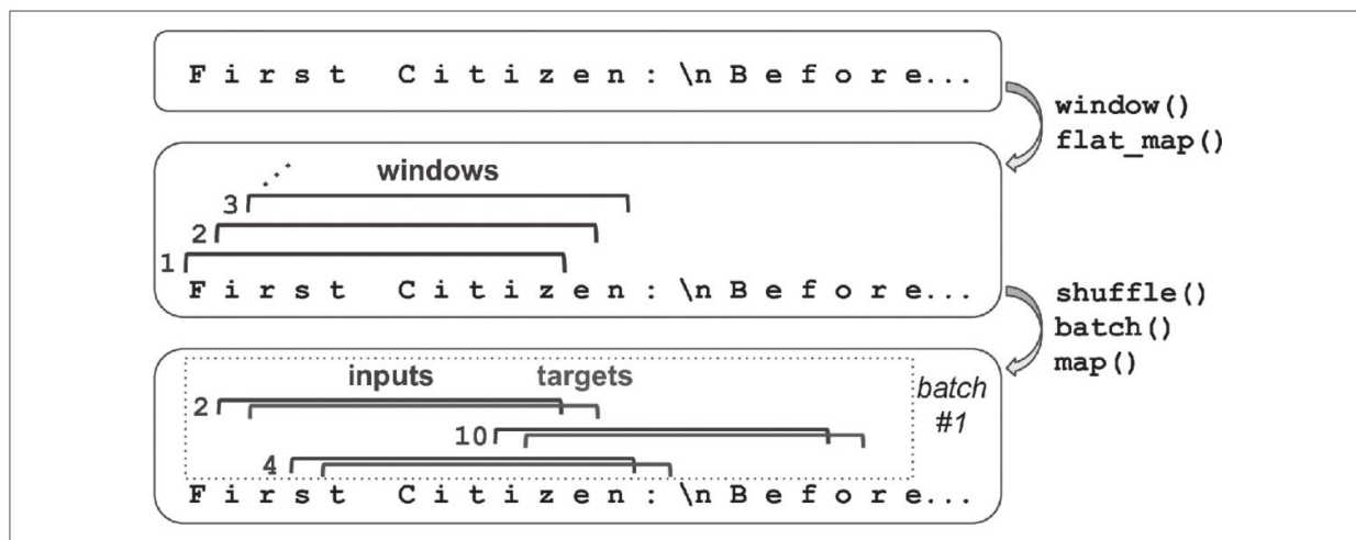
图16-1：准备随机窗口的数据集
