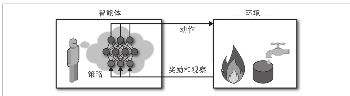
图18-2：使用神经网络策略进行强化学习
