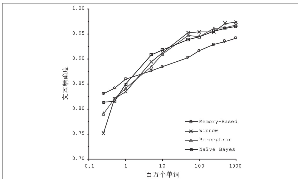
图1-20：数据与算法的重要性 [2]
