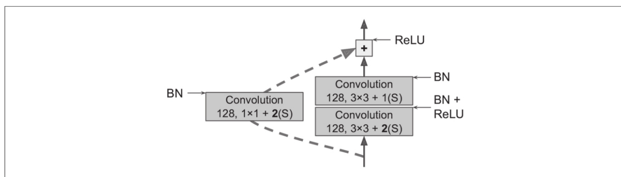
图14-18：改变特征图大小和深度的跳过连接
