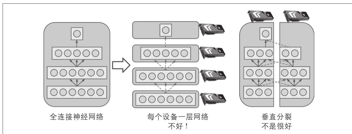
图19-15：划分一个完全连接的神经网络
