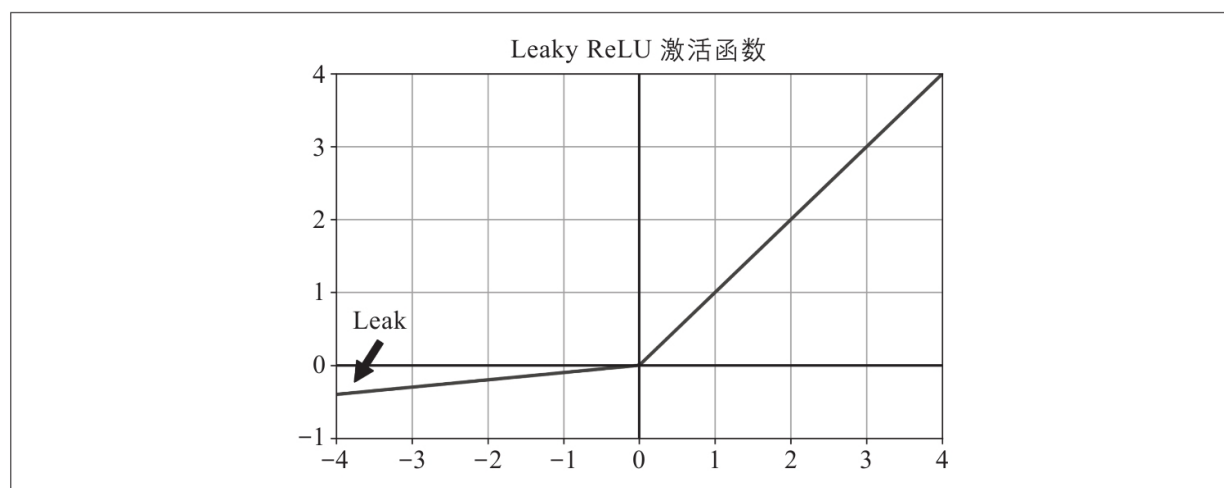
图11-2: Leaky ReLU: 与ReLU类似，对负值有一个小斜率
