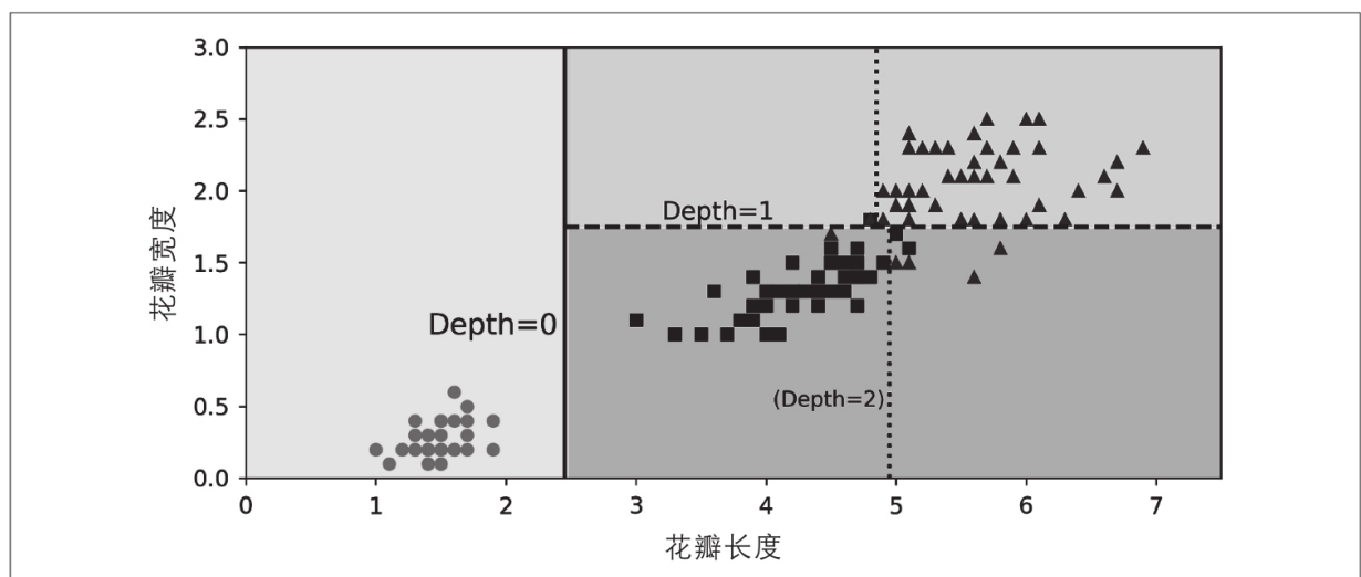
图6-2：决策树决策边界
