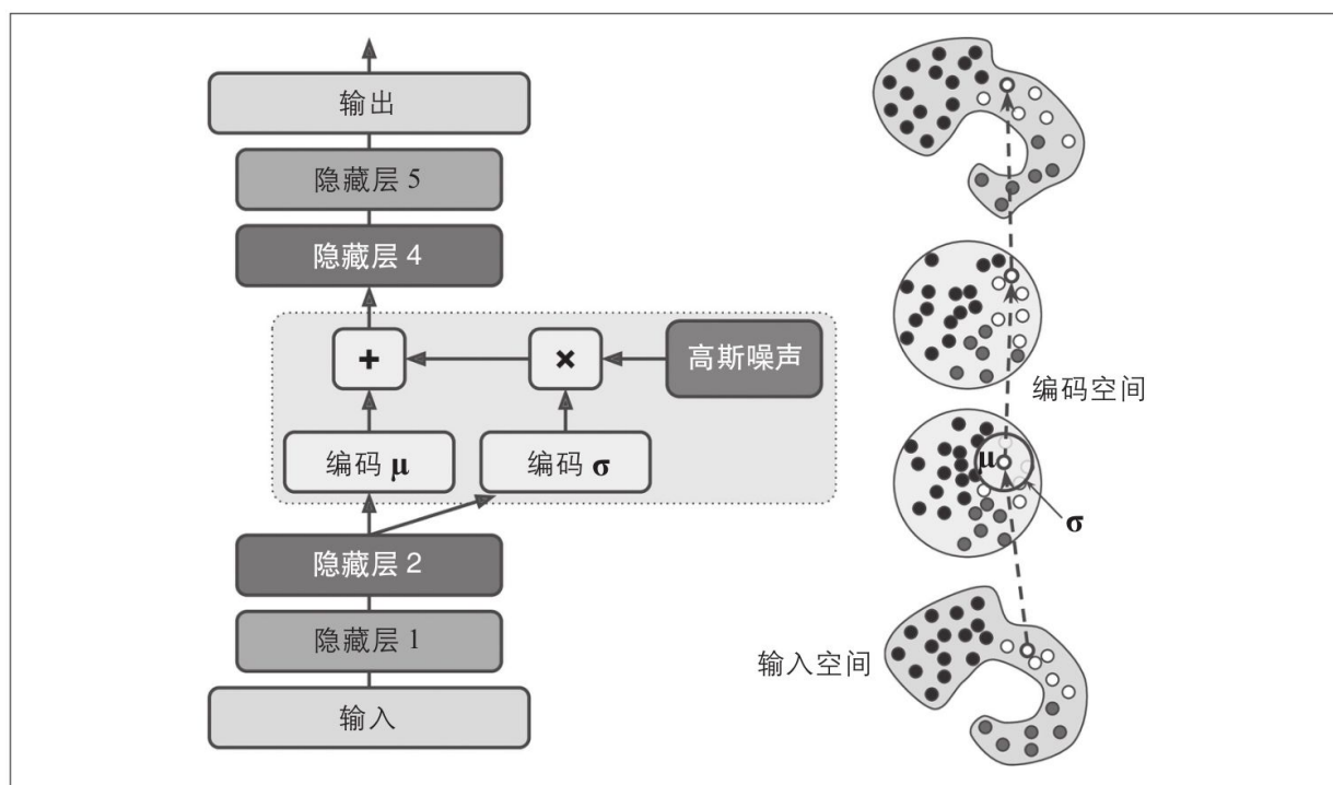
图17-12：变分自动编码器（左）和通过它的一个实例（右）
