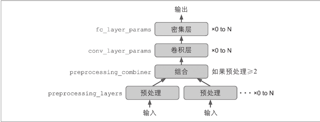
图18-14：编码网络的架构
