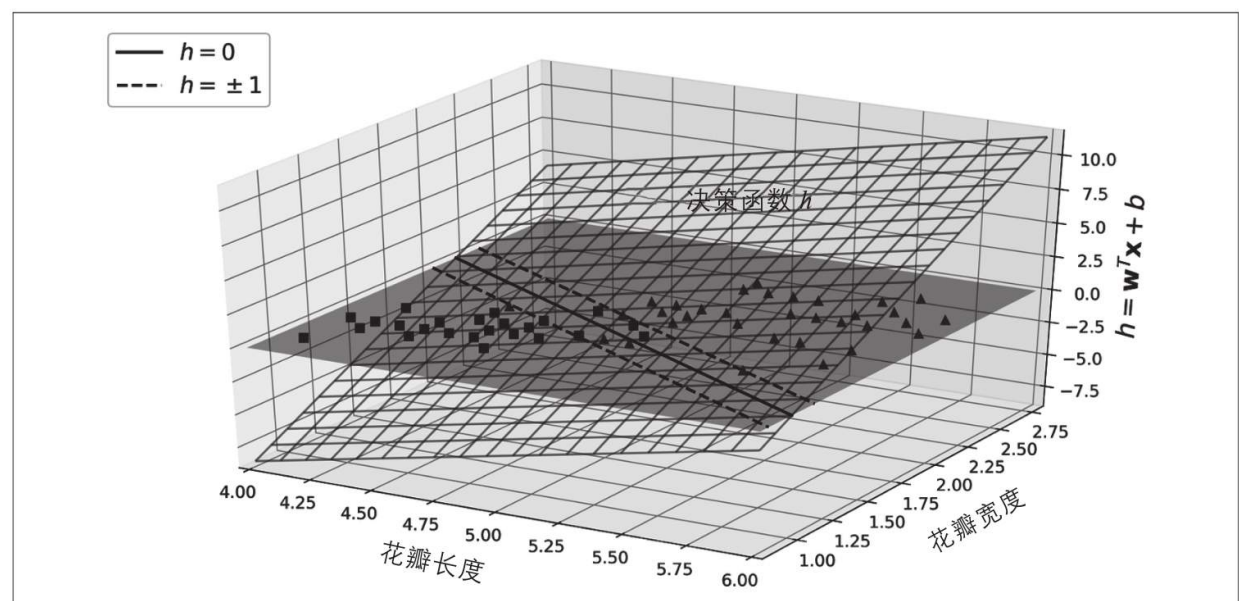
图5-12：鸢尾花数据集的决策函数
