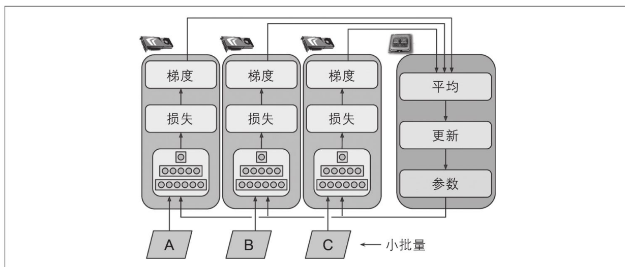
图19-19：具有集中参数的数据并行
