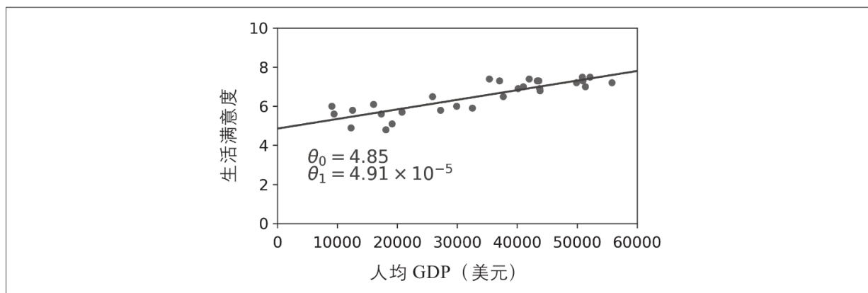
图1-19：最拟合训练数据的线性模型
