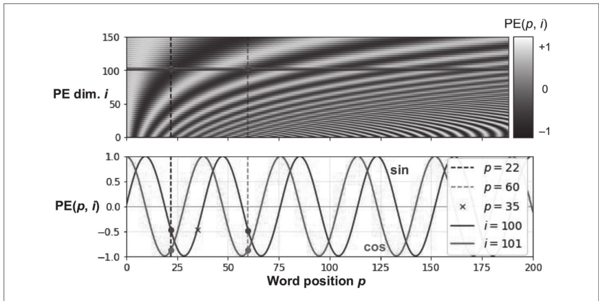
图16-9：正弦/余弦位置嵌入矩阵（转置，上），关注两个i值（下）
