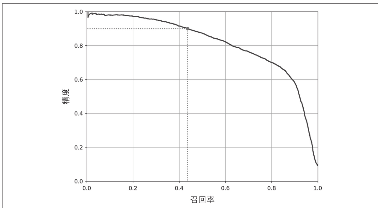
图3-5：精度与召回率
