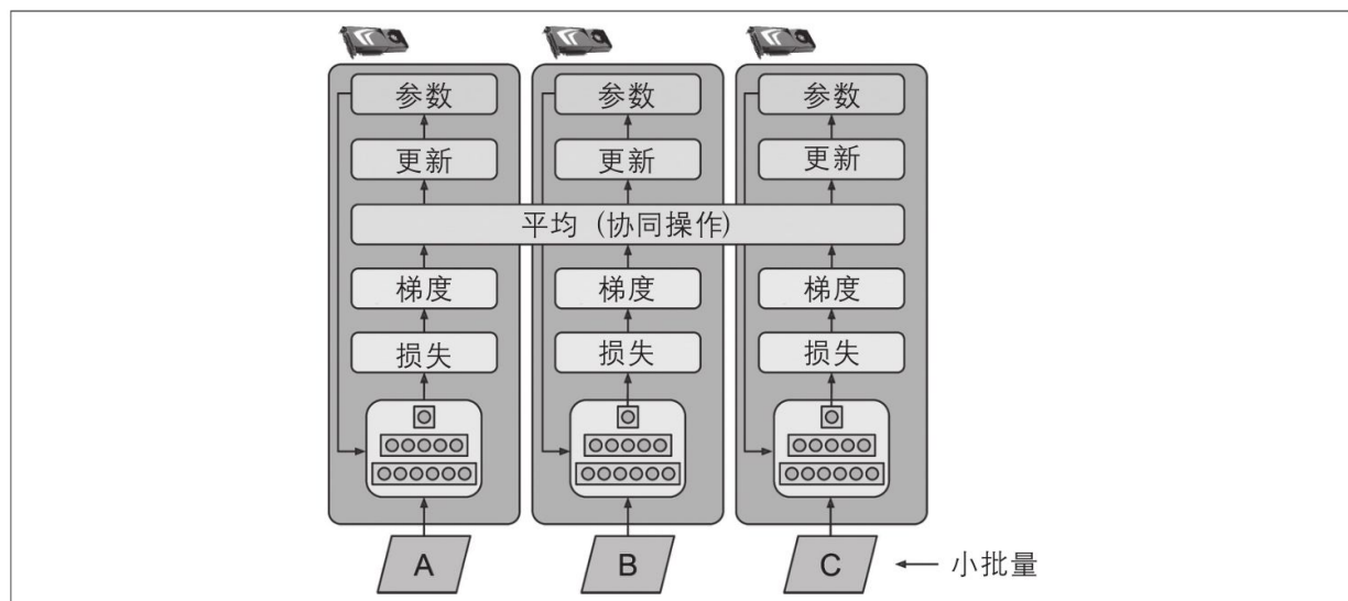
图19-18：使用镜像策略的数据并行
