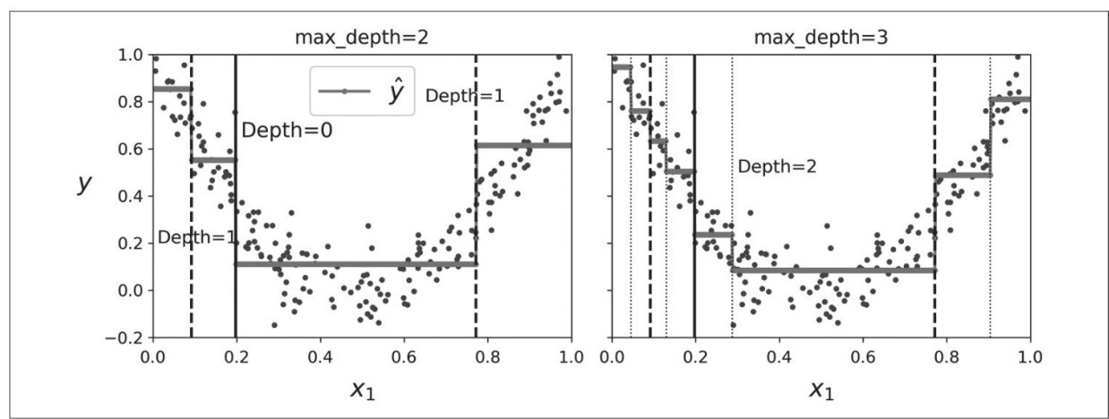
图6-5：两种决策树回归模型的预测
