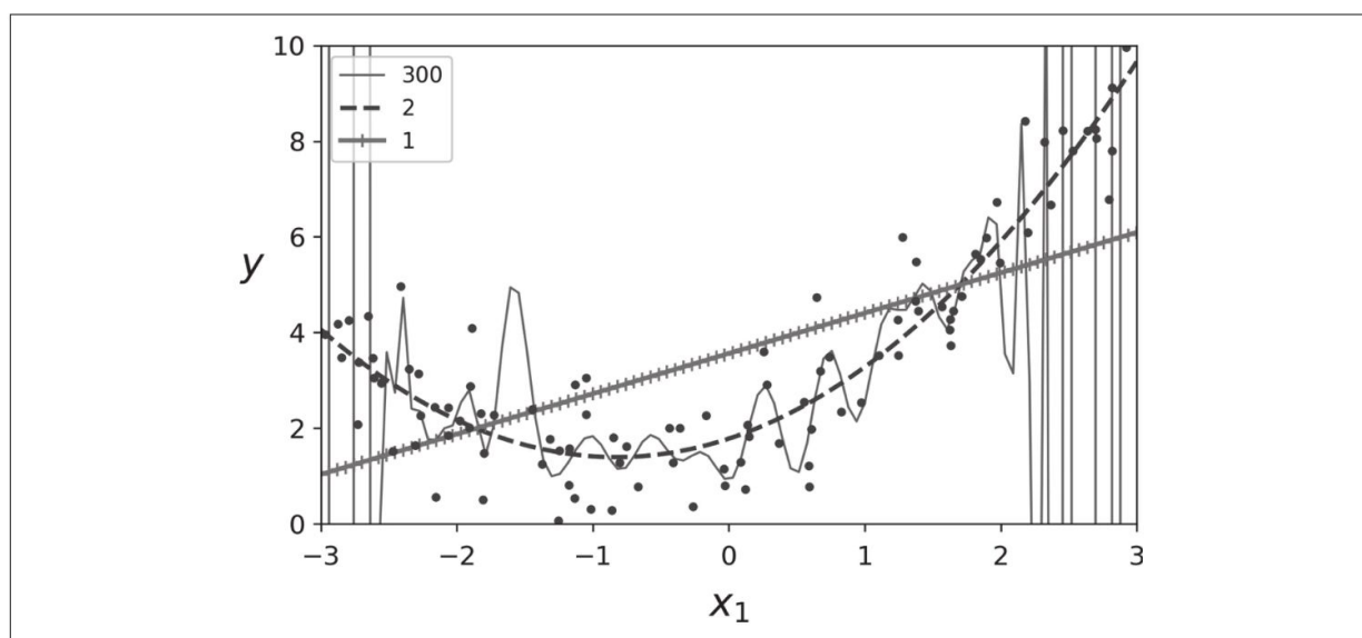
图4-14：高阶多项式回归
