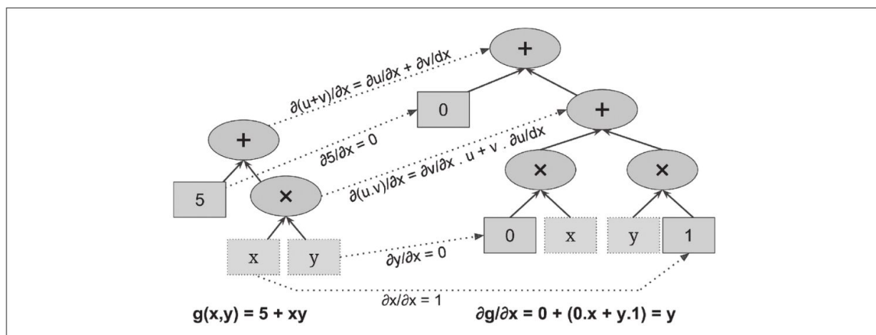
图D-1：前向模式自动微分
