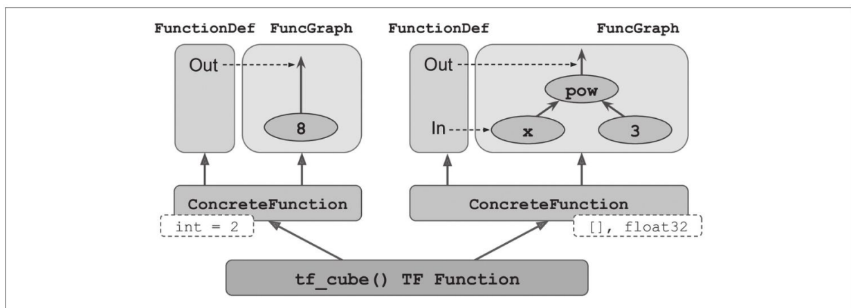
图G-1： tf_cube() TF函数及其具体函数和它们的函数图
