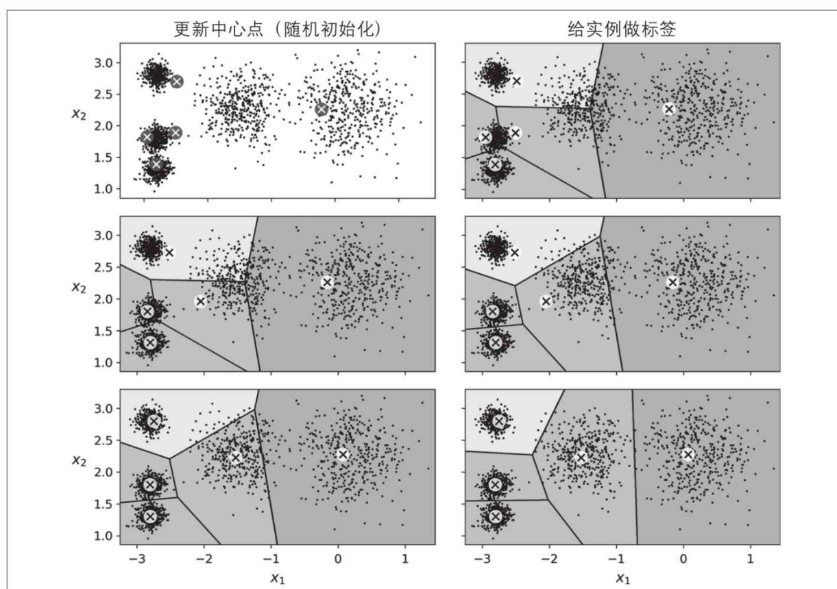
图9-4：K-Means算法
