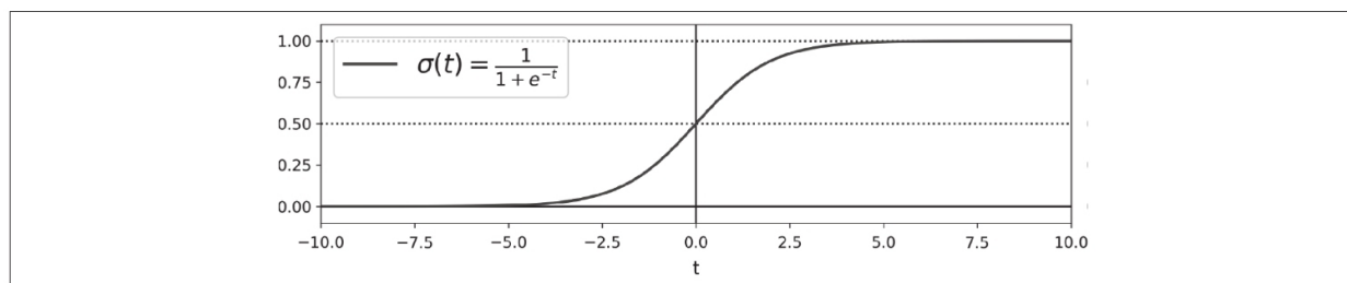
图4-21：逻辑函数
