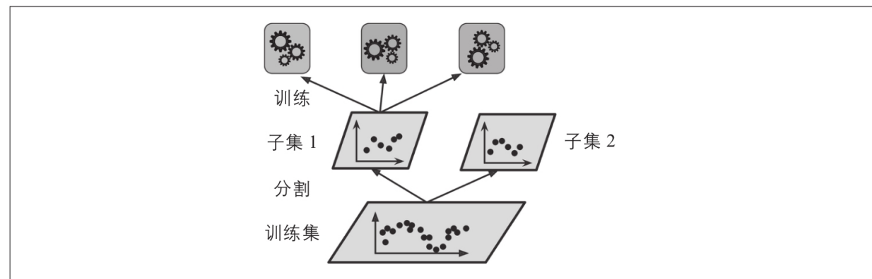
图7-13：训练第一层
