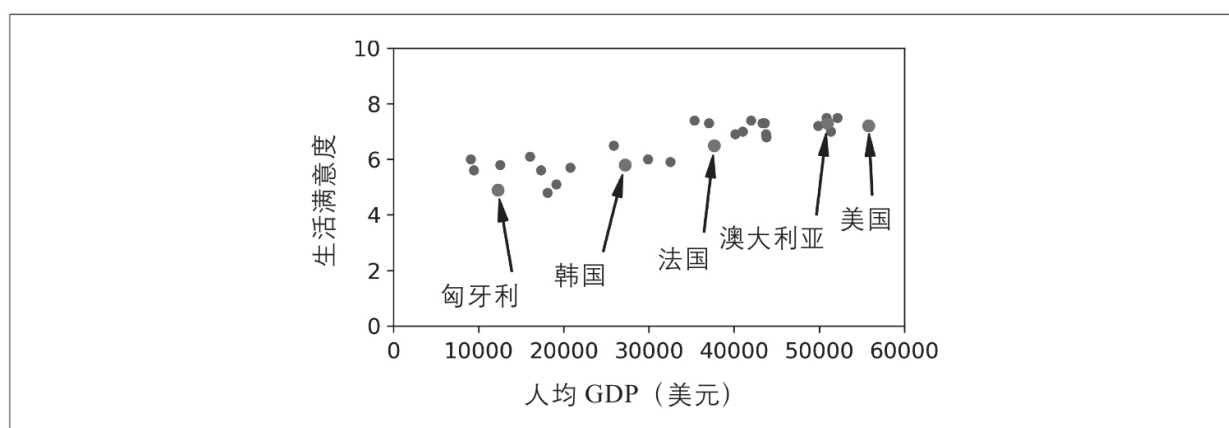
图1-17：趋势图
