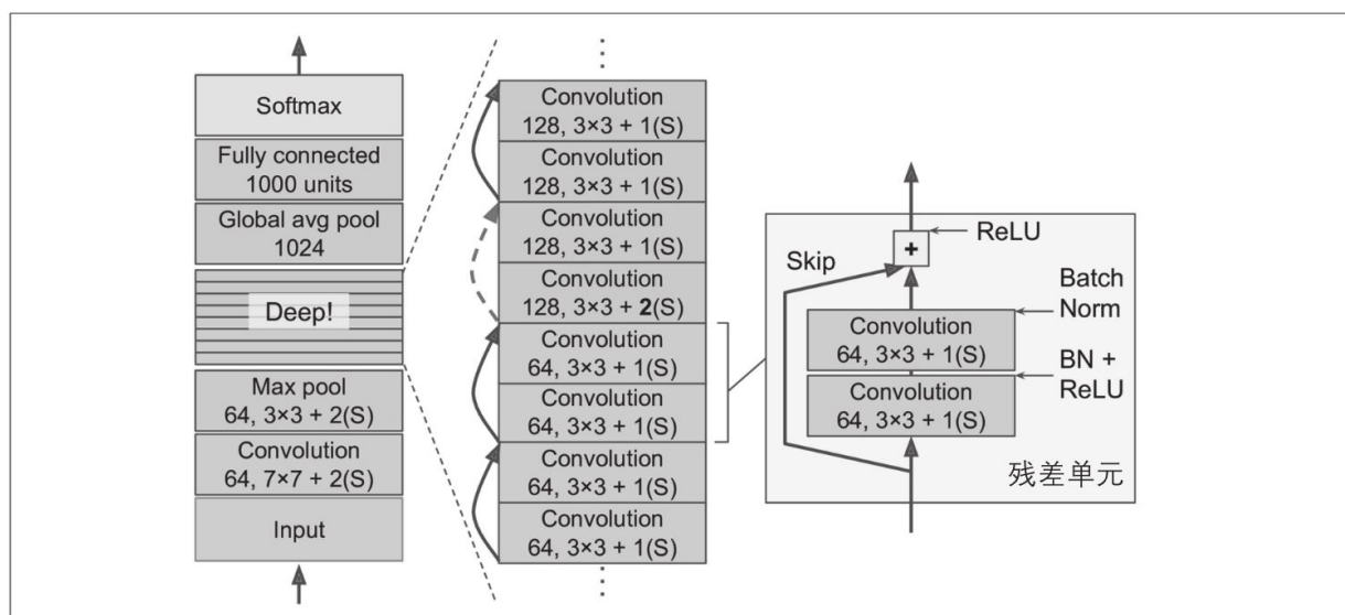
图14-17：ResNet架构
