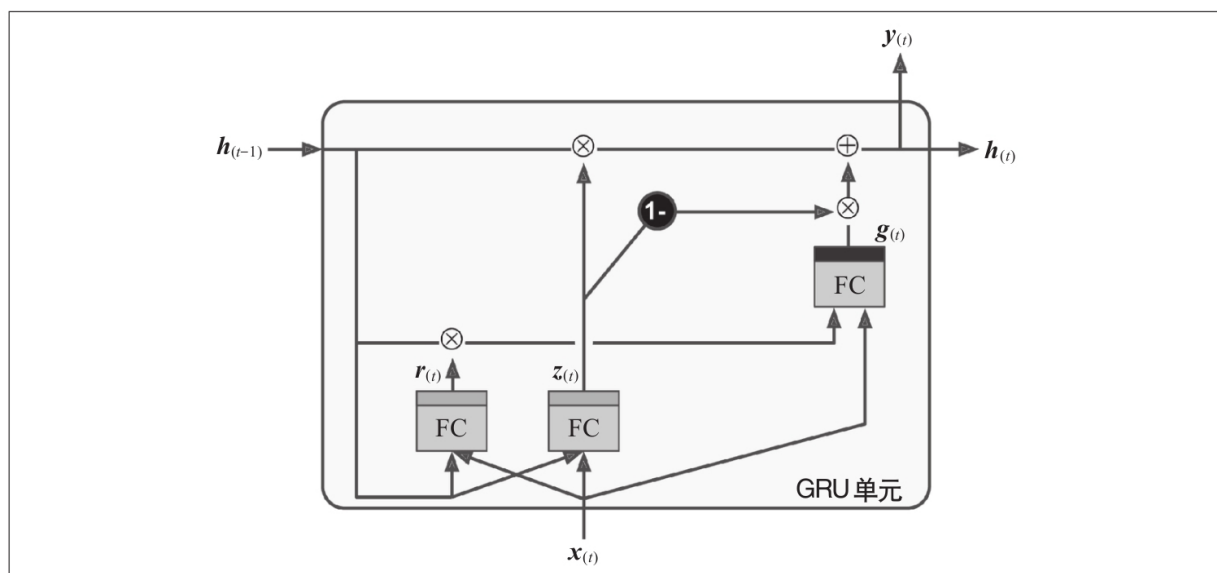
图15-10：GRU单元
