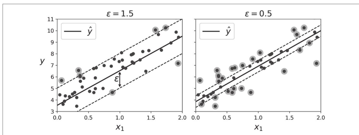
图5-10：SVM回归
