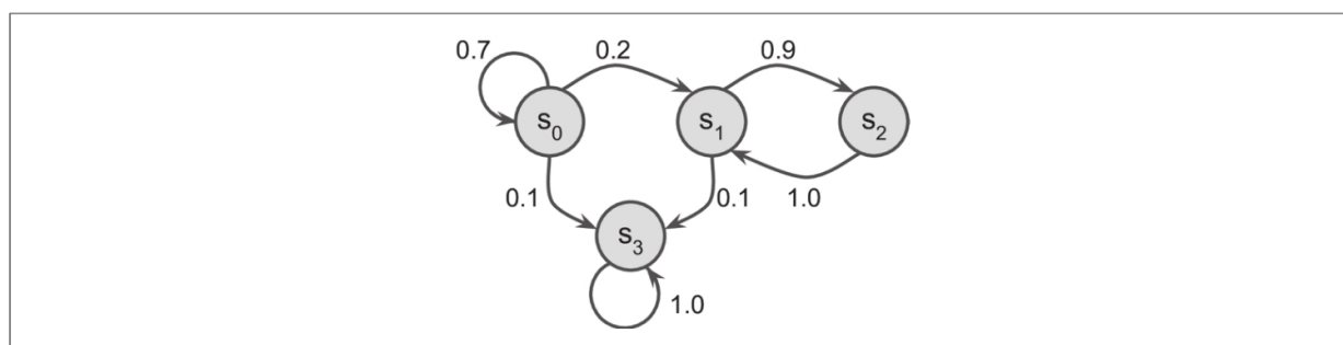
图18-7：马尔可夫链的示例
