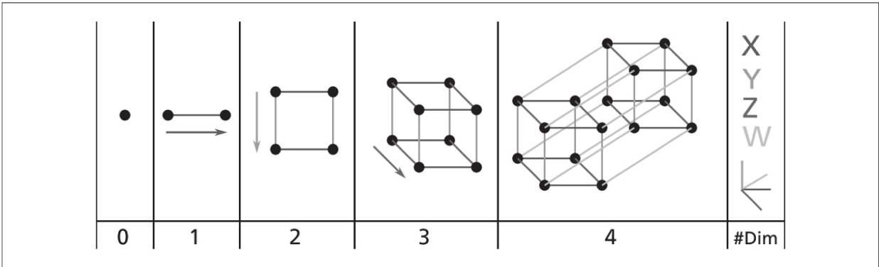
图8-1：点、线段、正方形、立方体和网格（零维至四维超立方体） [2]
