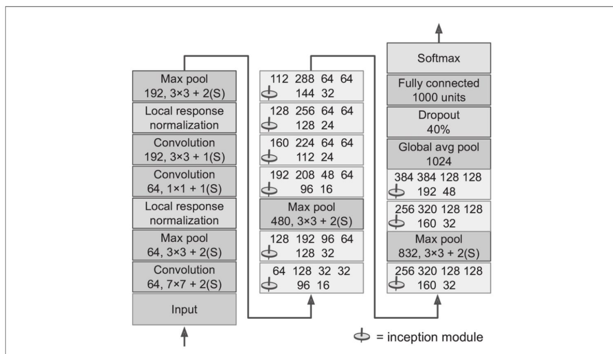
图14-14：GoogLeNet架构
