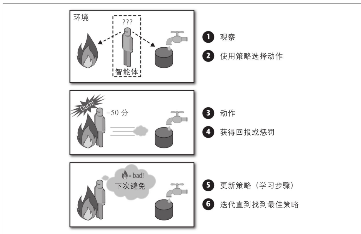
图1-12：强化学习
