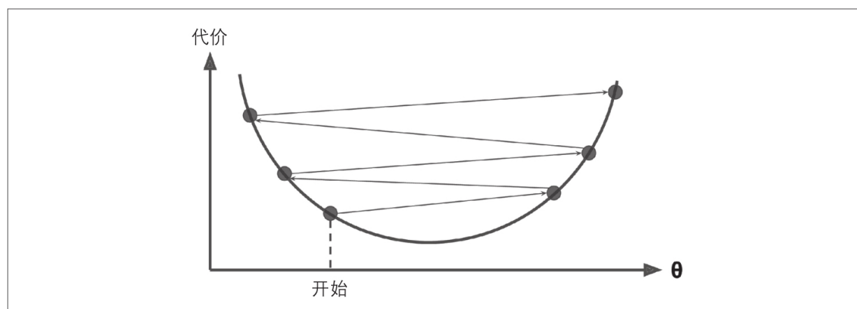
图4-5：学习率太高
