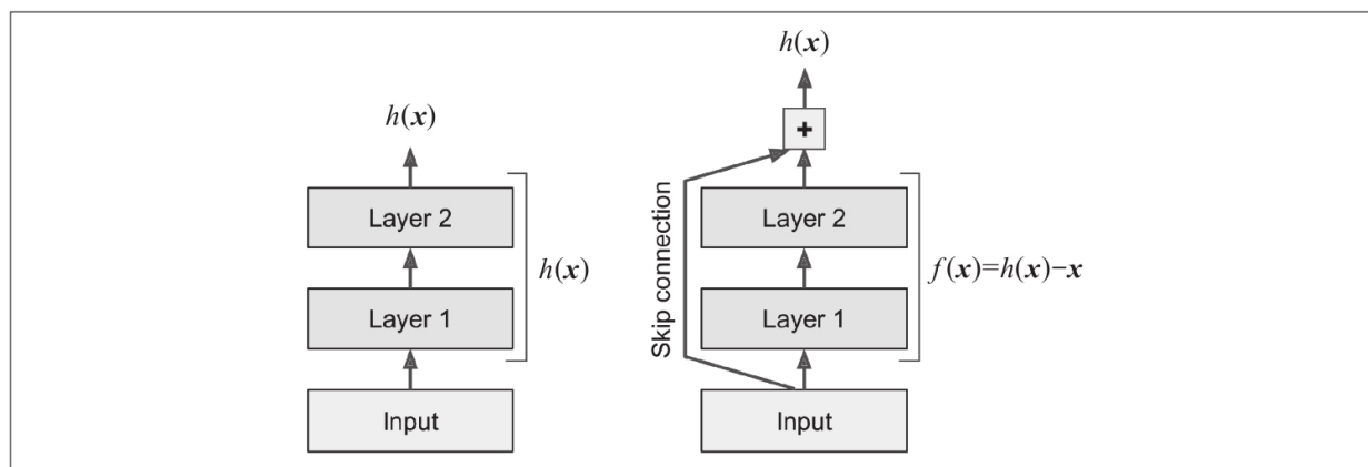
图14-15：残差学习
