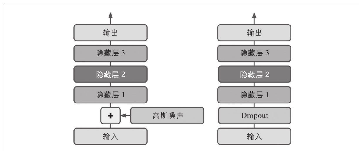
图17-8：具有高斯噪声（左）或dropout（右）的去噪自动编码器
