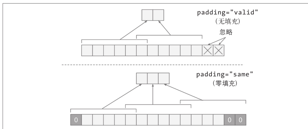
图14-7：Padding为“SAME”或“VALID”（输入宽度为13，滤波器宽度为6，步幅为5）
