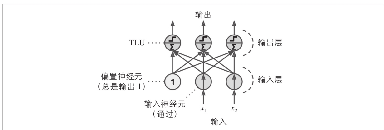
图10-5：具有两个输入神经元、一个偏置神经元和三个输出神经元的感知器架构
