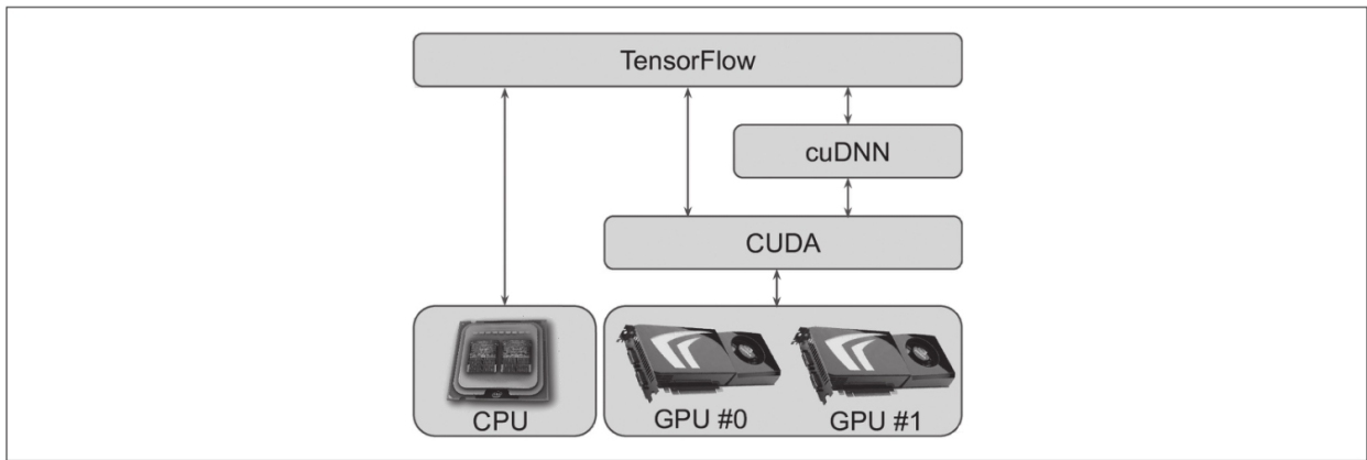
图19-10：TensorFlow使用CUDA和cuDNN来控制GPU和加速DNN
