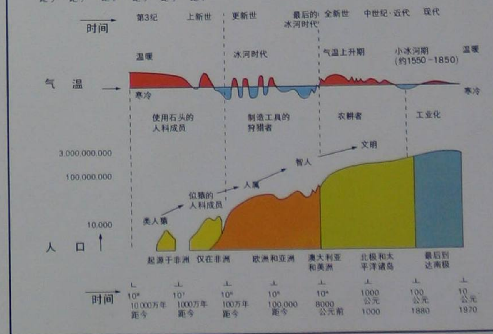
3 气候变迁和人口的增长 下图的对数尺度，标明更新世时期人口及气候的变化。这个真实的时间曲线表简要地说明近两百年内人口爆炸性增长的情况。
